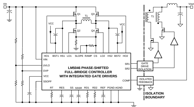
简化的相移全桥电源转换器
