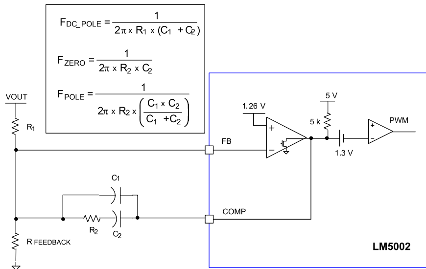
图 7-1. Type II Compensator
