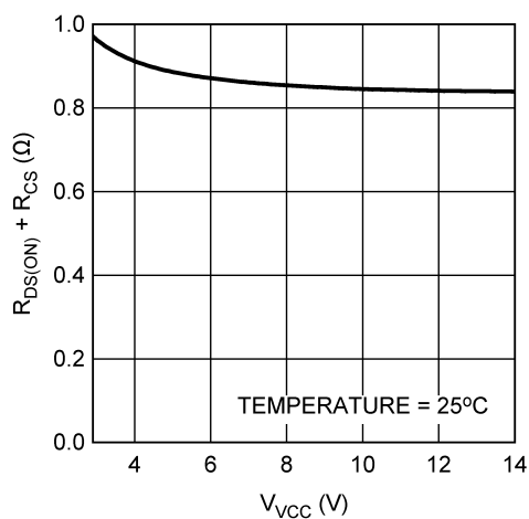
图 6-5. R_{DS(ON)} vs V_{CC}
