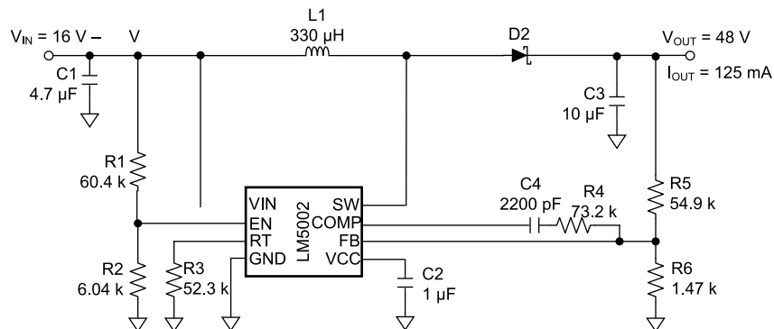
图 8-7. Boost Schematc
