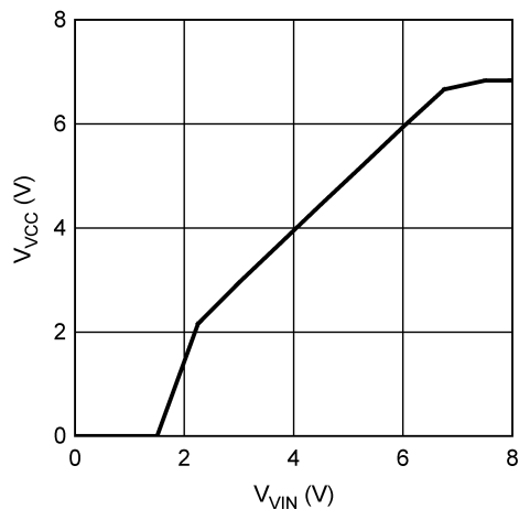
图 6-4. V_{CC} vs V_{IN}
