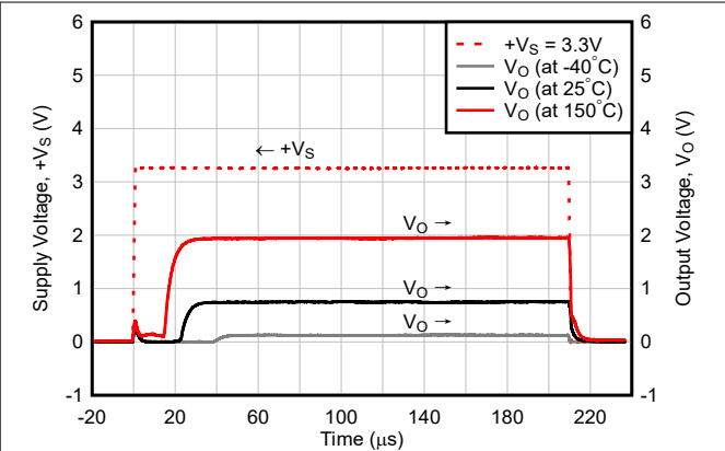
图 8-4. +V_S = 3.3V 阶跃时的启动响应（当 t_r = 1\mu s 、无 C_{Load} 和 C_{By-pass} 时）
