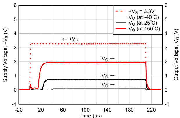
图 6-30. +V_S = 3.3\text{V} 阶跃时的启动响应 (当 t_r = 1\ \mu\text{s} 、无 C_{\text{Load}} 和 C_{\text{By-pass}} 时)
