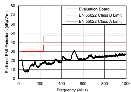
辐射发射图
