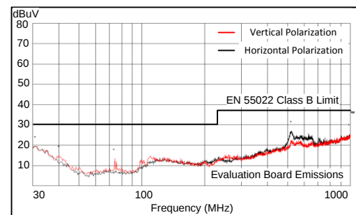
辐射发射图
