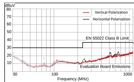
辐射发射图
