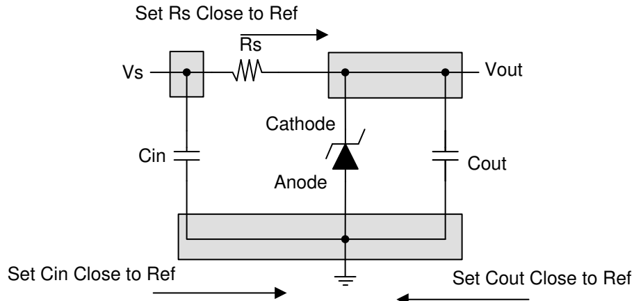
图 8-8. 布局建议
