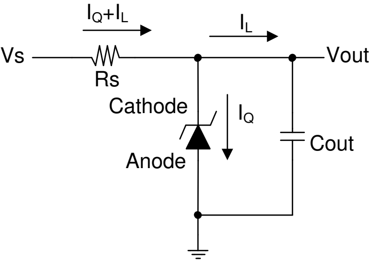
图 8-1. 并联稳压器原理图
