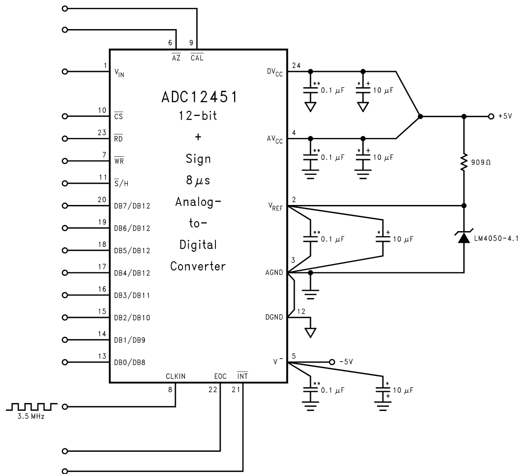
图 8-3. LM4050-N-4.1 的额定 4.096 击穿电压可提供 ADC12451 1mV/LSB
