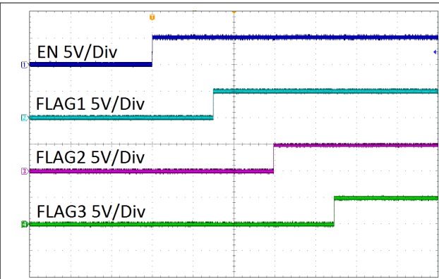
图 8-2. LM3880MF-1AB 的电源序列发生器
