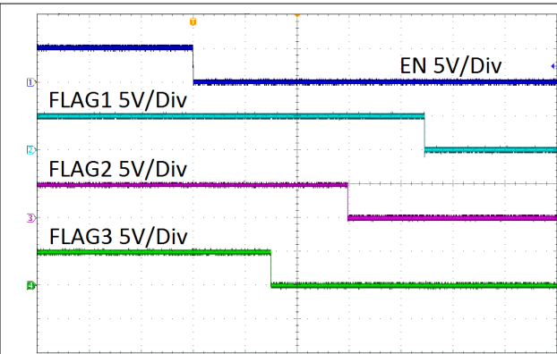
图 8-3. LM3880MF-1AB 的断电序列
