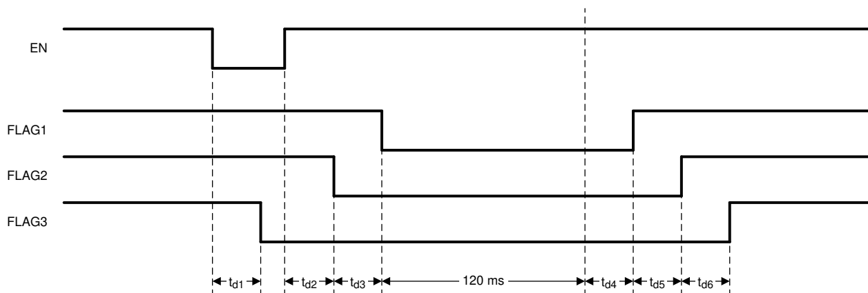
图 7-4. 不完整下电序列
