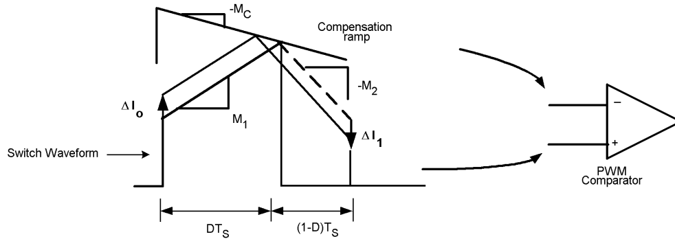
图 6-3. 补偿斜坡可避免次谐波振荡
