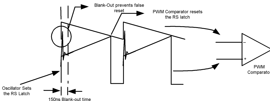
图 6-1. PWM 比较器的基本运行
