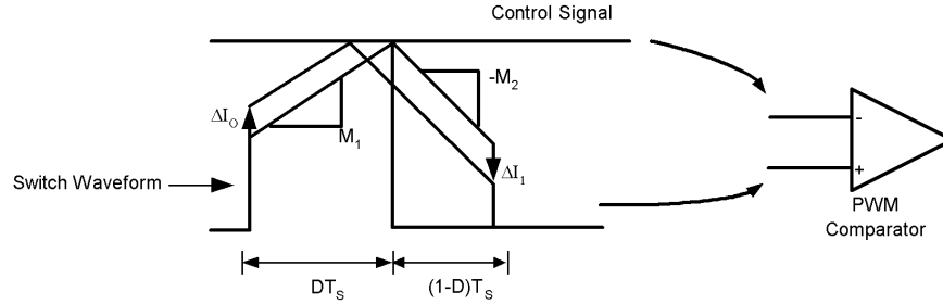
图 6-2. D>0.5 时的次谐波振荡
