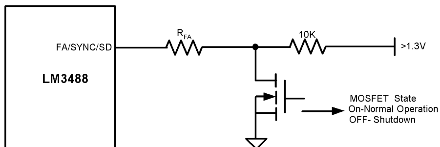
图 6-8. 频率调节模式下的关断运行
