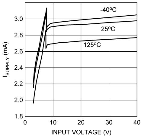
图 5-3. I_{Supply} 与 V_{IN} 间的关系
