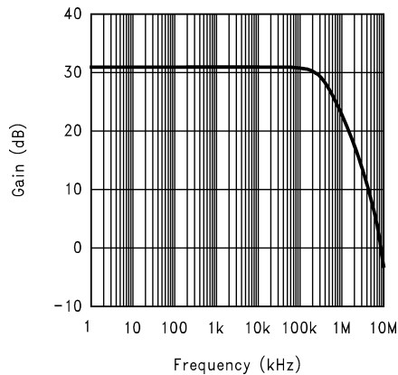
图 5-13. 误差放大器增益
