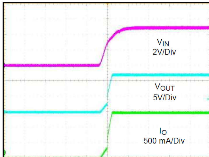
图 7-6. 典型启动波形 ( 水平标准 : 10ms/DIV )
