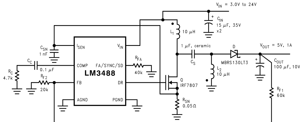
典型的 SEPIC 转换器
