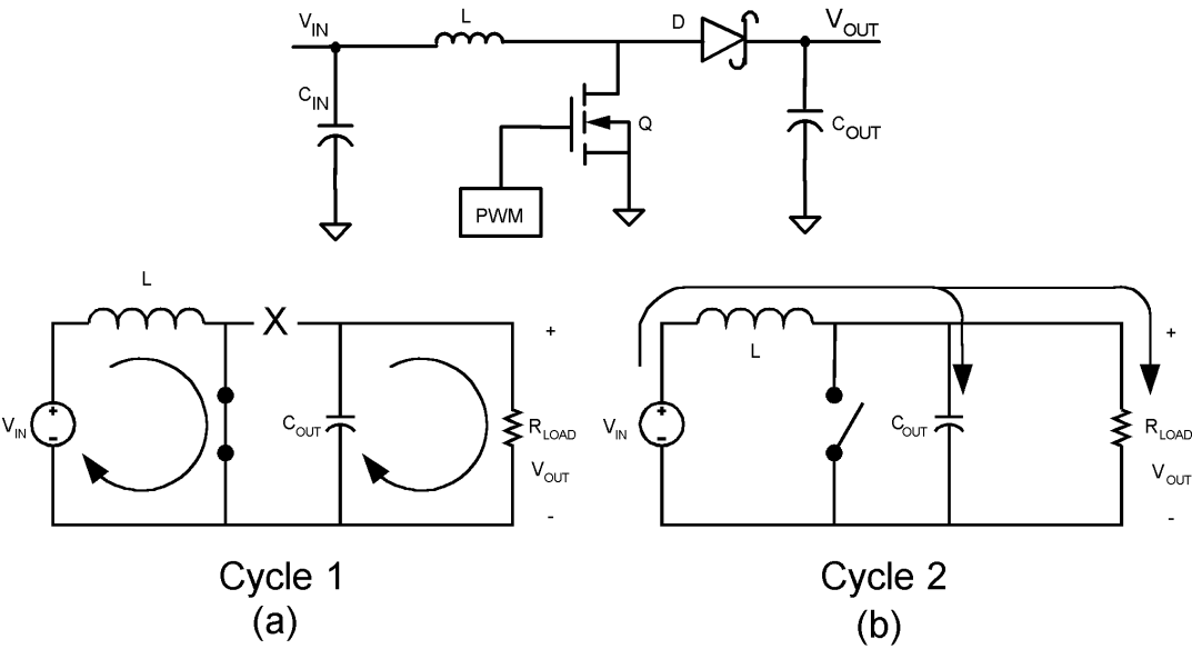
图 7-2. 升压转换器简化图 (a) 第一个运行周期 (b) 第二个运行周期
