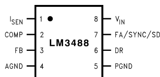
图 4-1. 8 引脚 D8V 封装 (顶视图)
