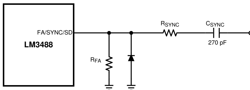
图 6-10. 频率调整或频率同步
