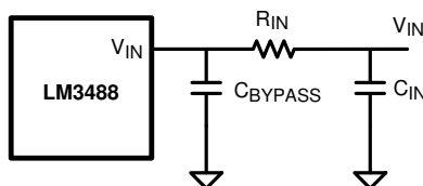
图 7-5. 降低 IC 输入噪声
