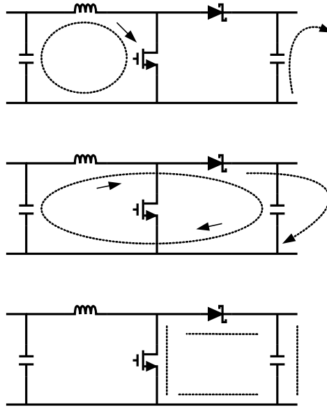
图 7-8. 升压应用中的电流流动
