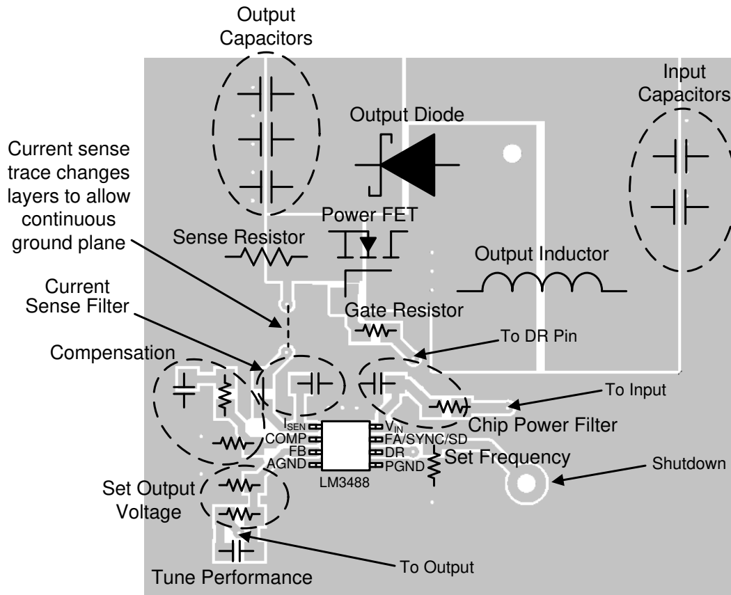
图 7-9. 使用 LM3488 的升压应用的布局示例
