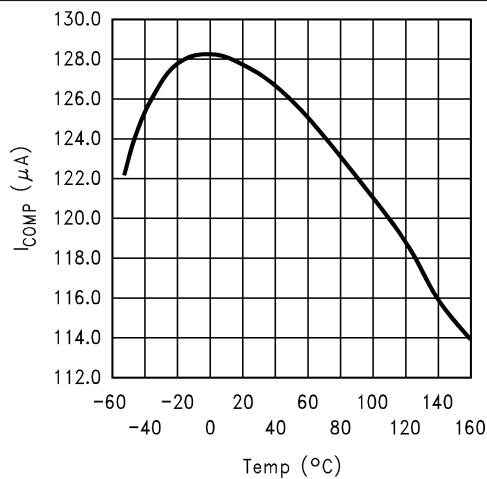
图 5-15. COMP 引脚拉电流与温度间的关系
