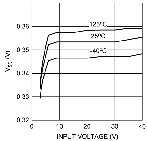
图 5-16. 短路保护与输入电压间的关系
