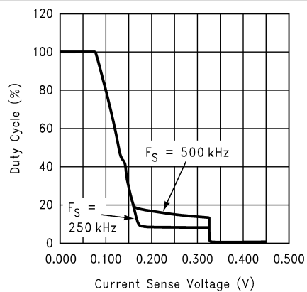
图 5-19. 电流检测电压与占空比间的关系
