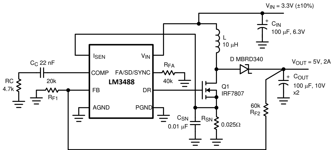
图 7-1. 典型高效升压转换器
