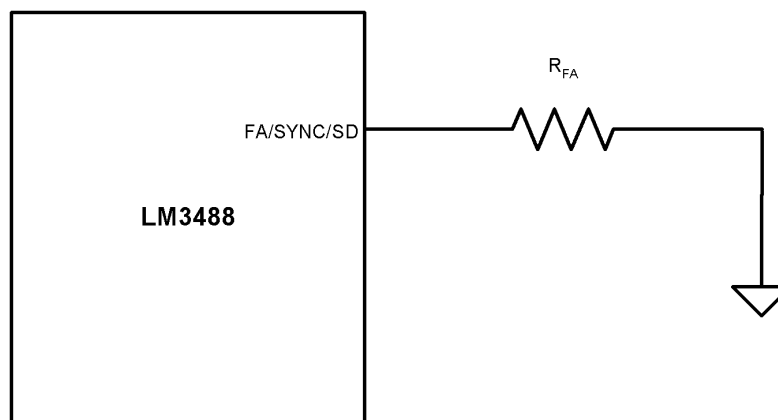
图 6-6. 频率调节
