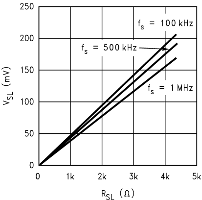
图 6-5. \Delta V_{SL} 与 R_{SL} 间的关系
