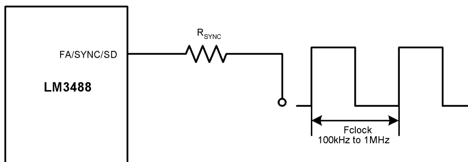
图 6-7. 频率同步
