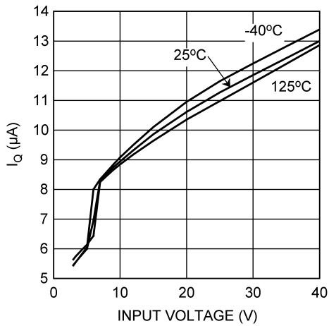
图 5-1. I_Q 与温度和输入电压间的关系
