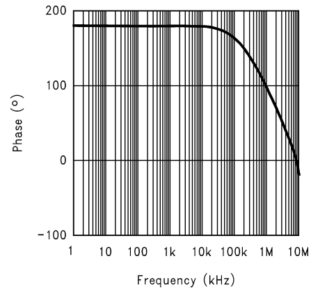
图 5-14. 误差放大器相位
