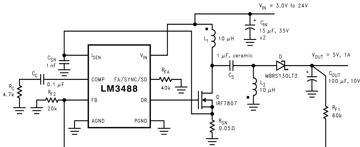
图 7-7. 典型的 SEPIC 转换器
