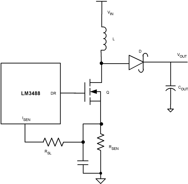
图 6-4. 增加补偿斜坡的斜率
