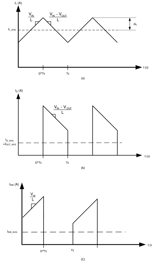
图 7-3. A. 电感器电流 B. 二极管电流 C. 开关电流
