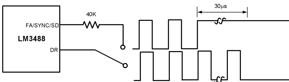
图 6-9. 同步模式下的关断运行
