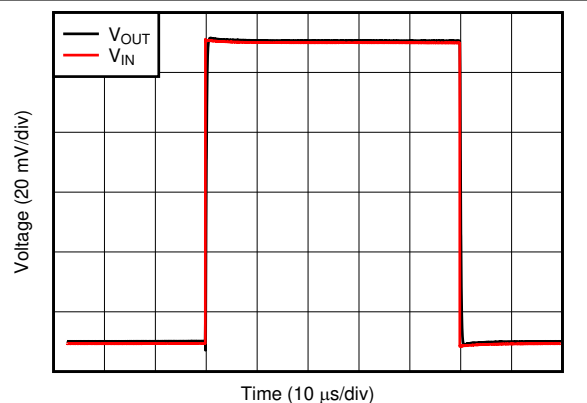
图 6-21. 无相位反转
