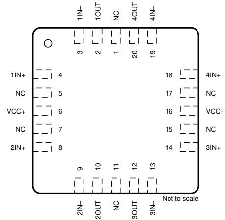
图 5-2. FK 封装， 20 引脚 LCCC (顶视图)
