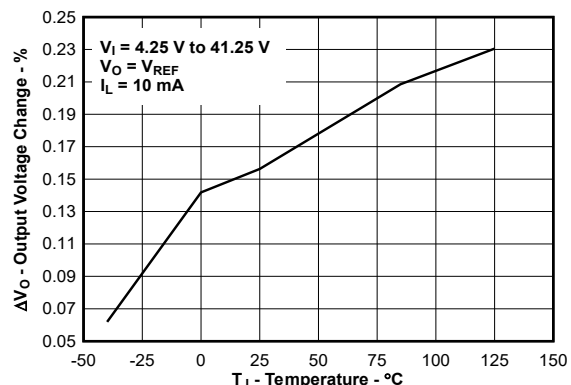
图 5-2. 线性调整率与温度间的关系 (新芯片)
