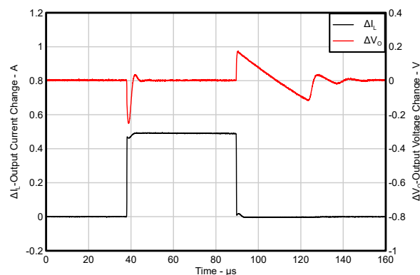
图 7-7. 负载瞬态响应与时间之间的关系 (新芯片)
