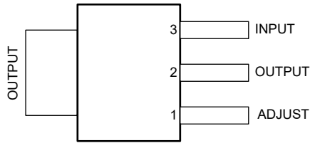
图 4-1. DCY 封装、4 引脚 SOT-223 (顶视图)
