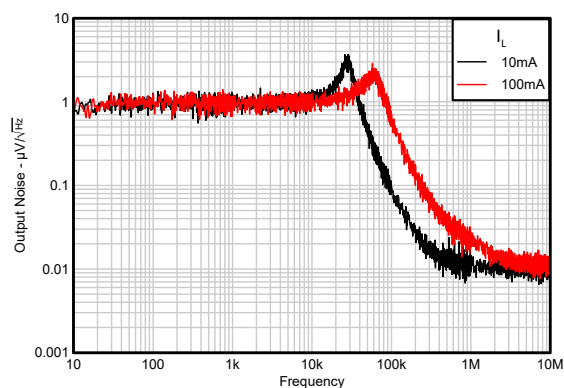
图 5-14. 输出噪声电压与输出电流间的关系 (新芯片)
