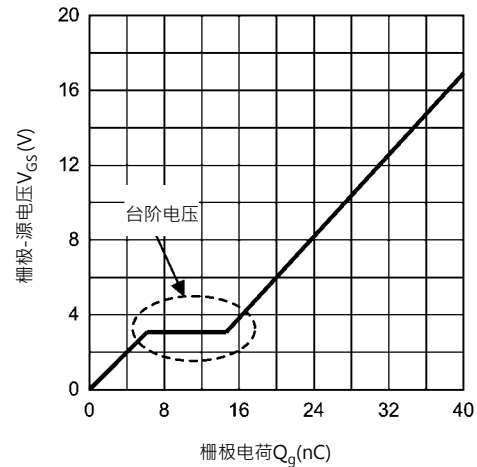
图3. 典型的MOSFET栅极电荷曲线
