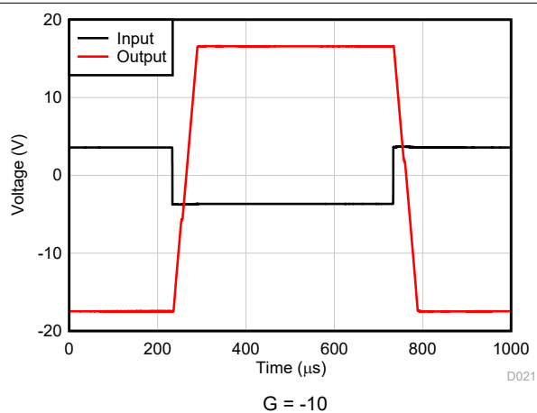
图 7-28. 过载恢复
