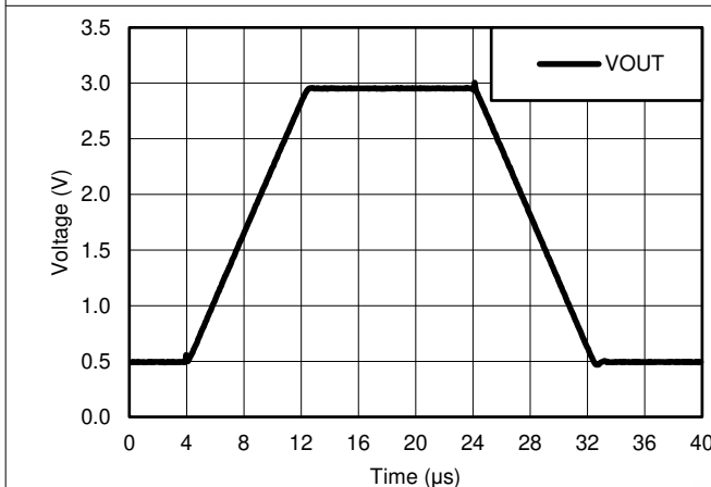
图 5-43. 电压跟随器大信号脉冲响应 (50pF)
