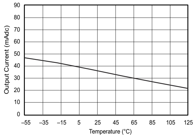
图 5-48. 拉电流限制
