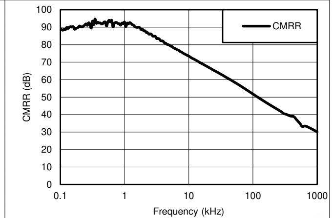
图 5-42. 共模抑制比与频率间的关系
