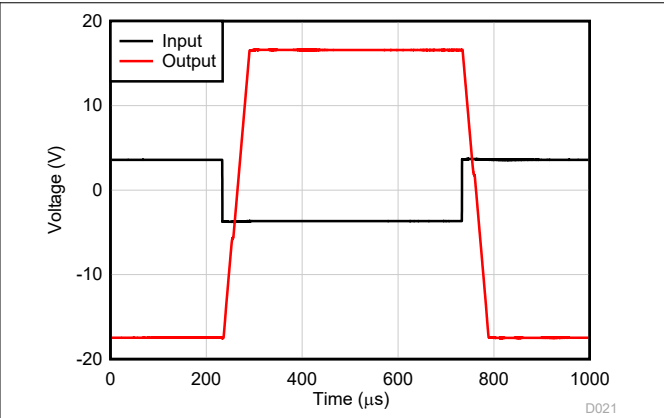
图 5-28. 过载恢复
