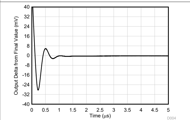
图 5-30. 小信号阶跃响应， G = -1
