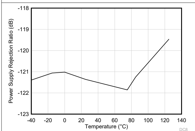
图 5-15. 电源抑制比与温度间的关系 (dB) V_S = 5\text{V} 至 36\text{V}
