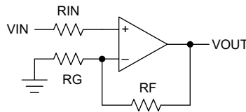
图 9-4. 同相配置的运算放大器原理图
