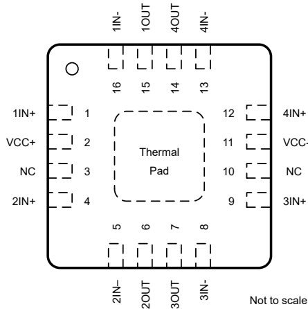
图 5-3. RTE 封装， 16 引脚 WQFN ( 顶视图 )
