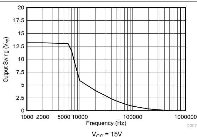
图 6-40. 最大输出摆幅与频率间的关系
