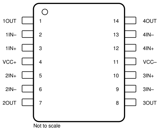
图 5-1. D、DB、J、N、NS、PW、W 封装， 14 引脚 SOIC、SSOP、CDIP、PDIP、SO、 TSSOP、CFP (顶视图)
