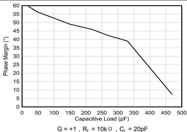
图 6-23. 相位裕度与容性负载间的关系
