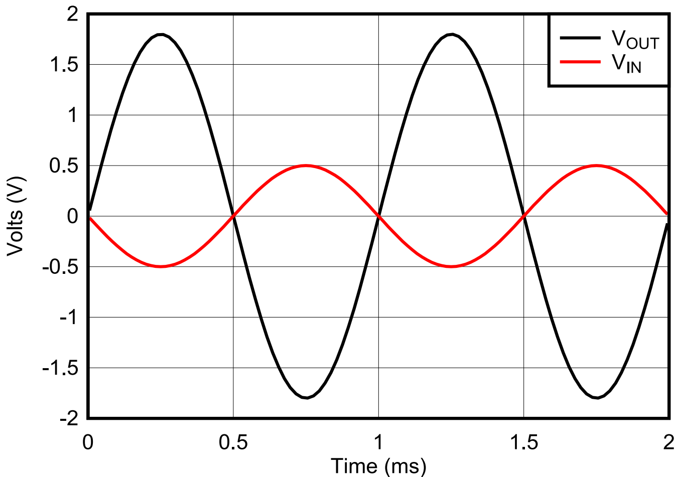
图 9-2. 反相放大器的输入和输出电压
