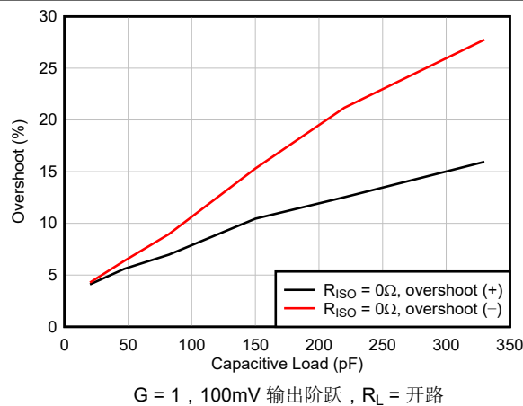
图 6-21. 小信号过冲与容性负载间的关系
