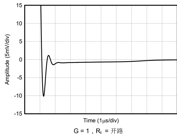
图 6-26. 小信号阶跃响应， G = 1
