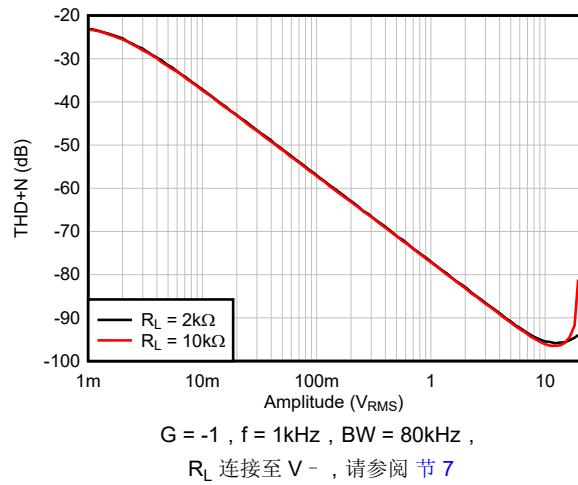
图 6-17. THD+N 与输出振幅间的关系， G = -1
