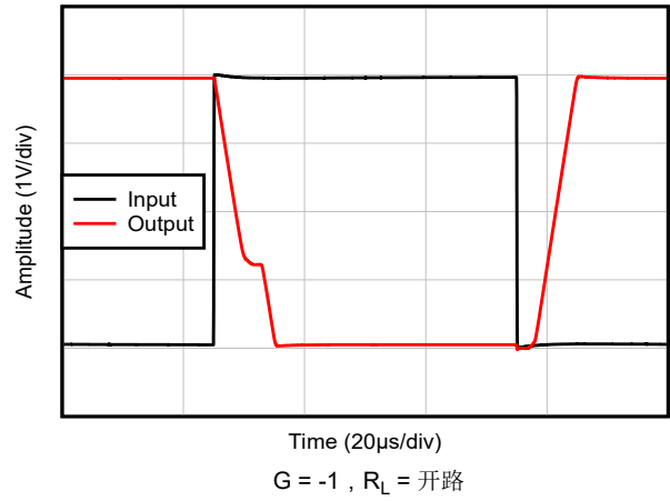
图 6-30. 大信号阶跃响应， G = -1
