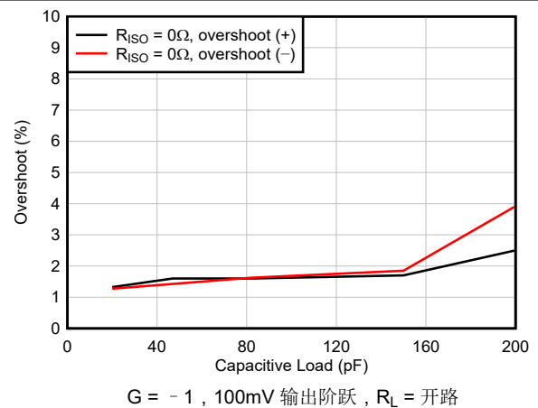
图 6-22. 小信号过冲与容性负载间的关系
