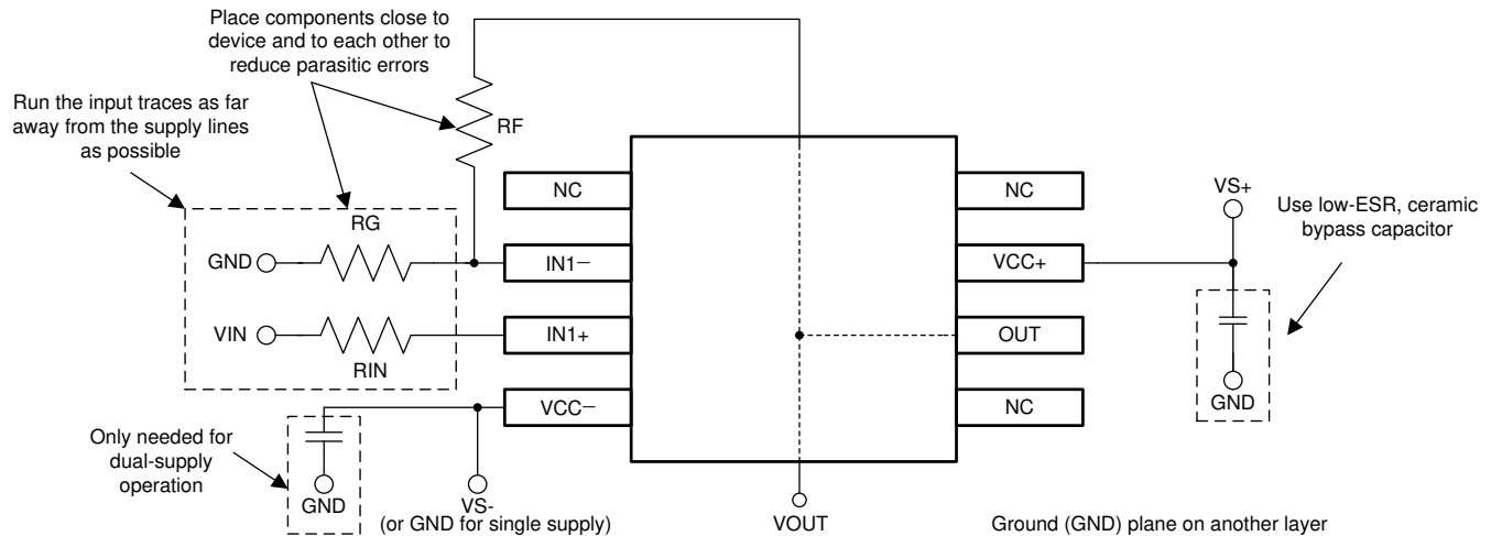
图 9-3. 同相配置的运算放大器电路板布局
