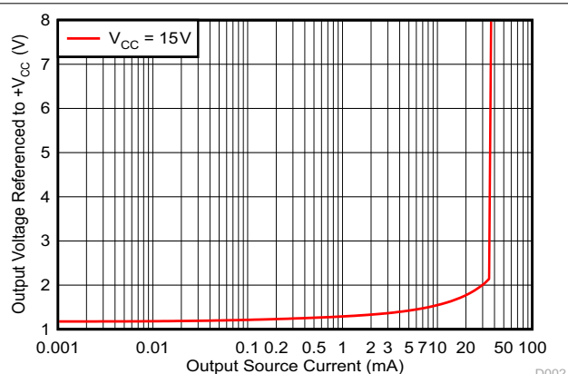
图 6-36. 输出拉电流特性
