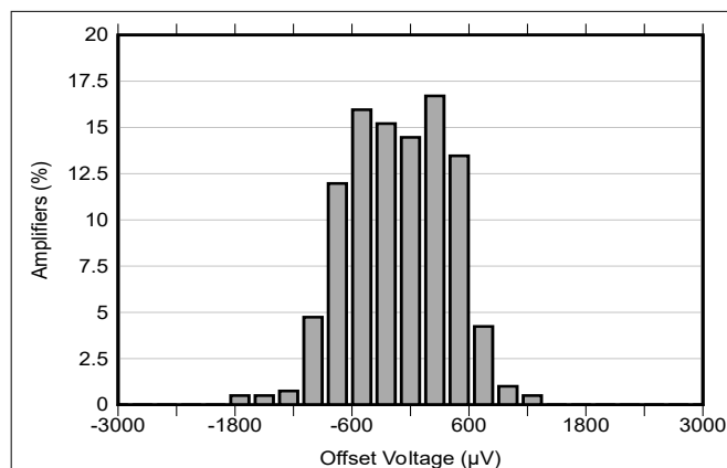
图 6-1. 失调电压产生分布
