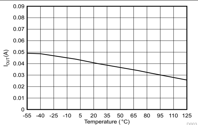
图 6-35. 输出灌电流特性
