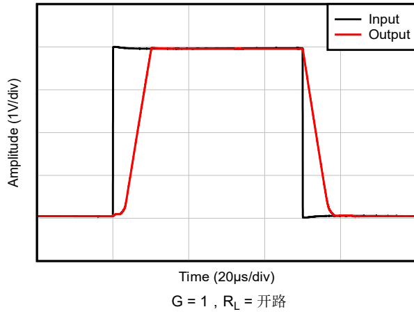
图 6-29. 大信号阶跃响应， G = 1
