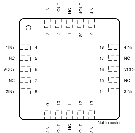
图 5-2. FK 封装, 20 引脚 LCCC (顶视图)
