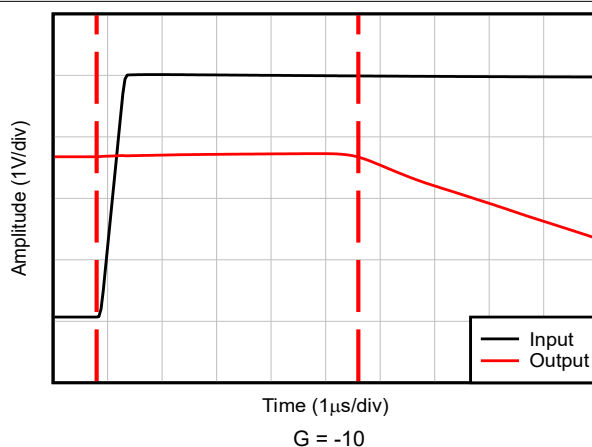
图 6-24. 过载恢复（正轨）
