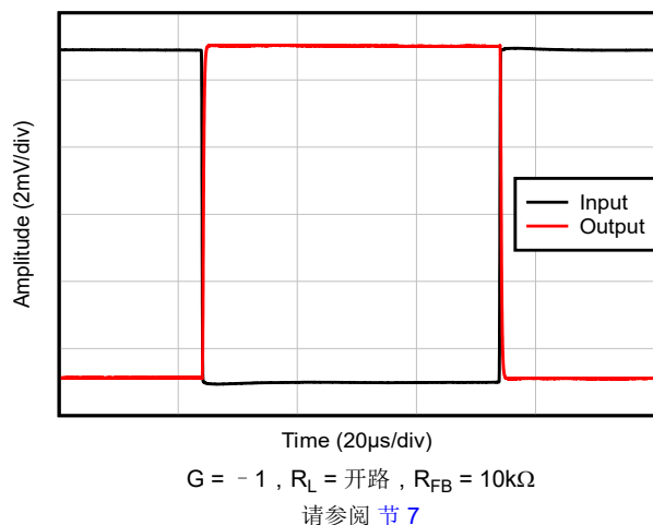
图 6-27. 小信号阶跃响应， G = -1
