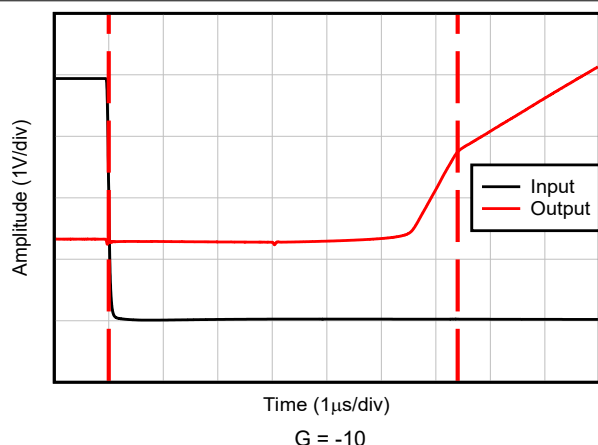
图 6-25. 过载恢复（负轨）
