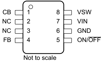
图 4-1. D 或 P 封装 8 引脚 SOIC 或 PDIP (顶视图)
