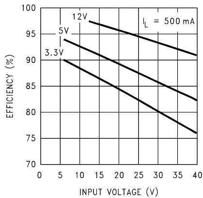
图 5-3. 效率
