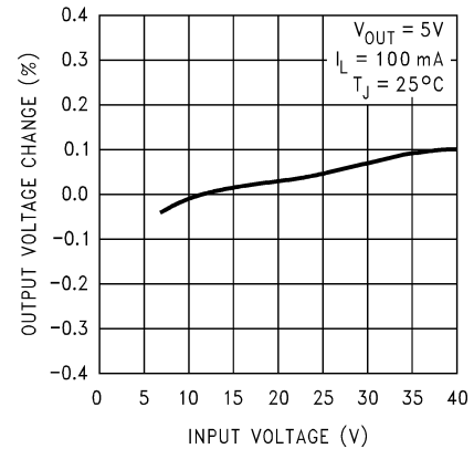
图 5-2. 线性调整率
