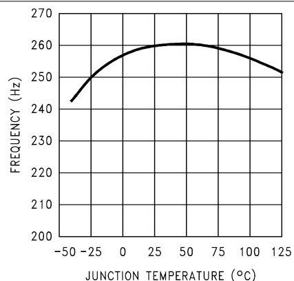
图 5-10. 开关频率
