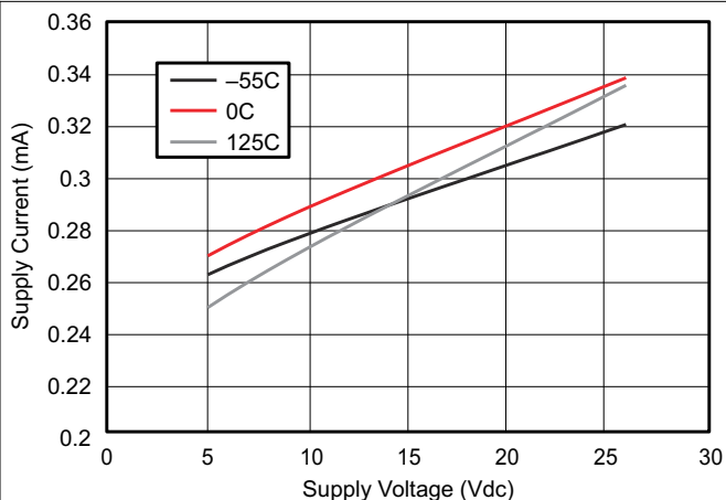
图 5-40. 电源电流与电源电压间的关系
