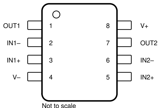
图 4-1. D、DDF、DGK、P、PS、PW 和 JG 封装 8 引脚 SOIC、SOT23-8、VSSOP、PDIP、SO、 TSSOP 和 CDIP 顶视图
