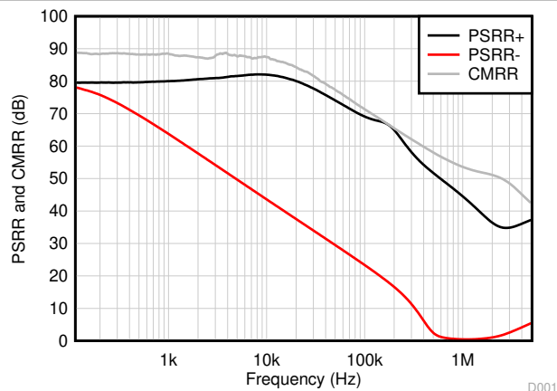
图 5-13. CMRR 和 PSRR 与频率间的关系
