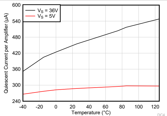
图 5-23. 静态电流与温度间的关系
