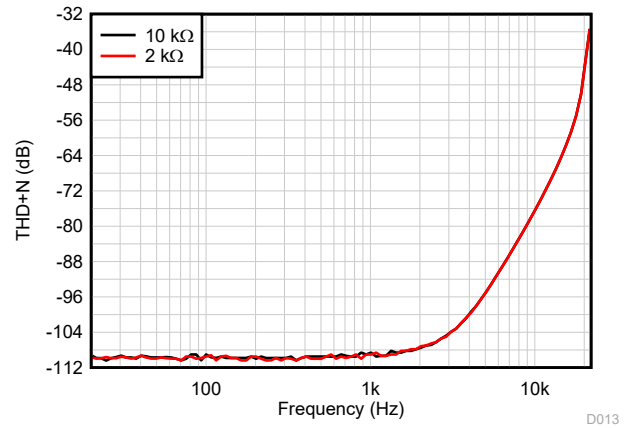
图 5-18. THD+N 比与频率间的关系， G = 1
