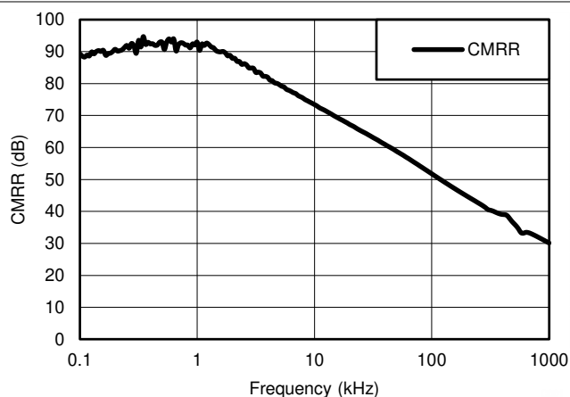
图 5-42. 共模抑制比与频率间的关系
