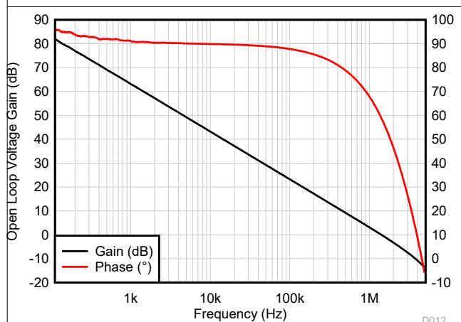
图 5-5. 开环增益和相位与频率间的关系
