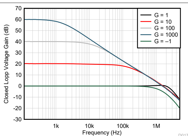
图 5-6. 闭环增益与频率间的关系
