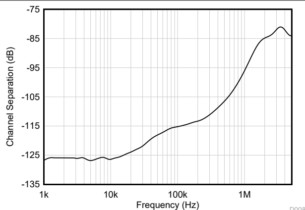
图 5-37. 通道隔离与频率间的关系
