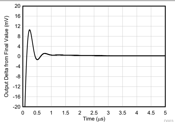
图 5-29. 小信号阶跃响应， G = 1
