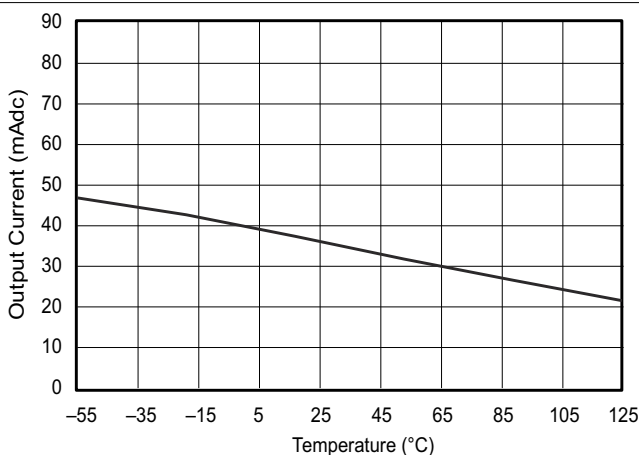
图 5-48. 拉电流限制
