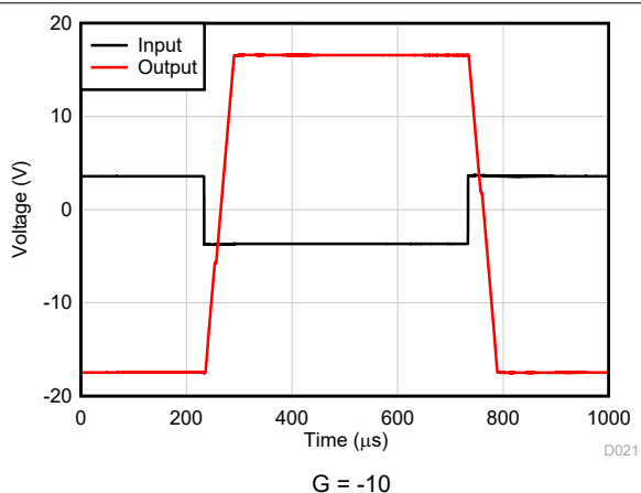
图 5-28. 过载恢复
