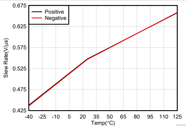
图 5-34. 压摆率与温度间的关系
