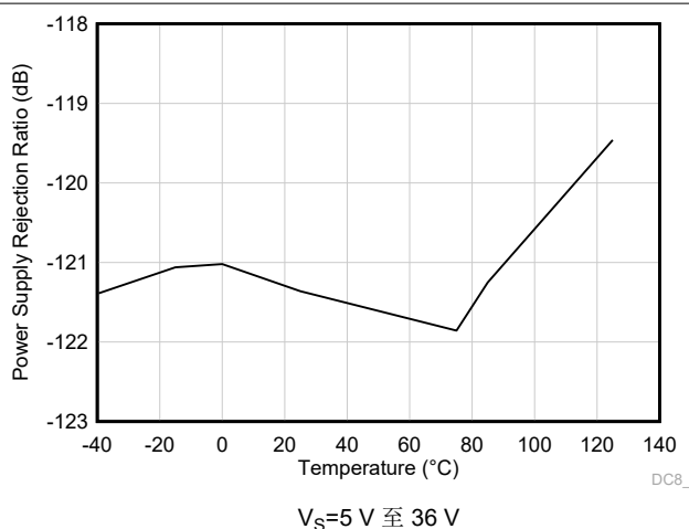
图 5-15. 电源抑制比与温度间的关系 (dB)
