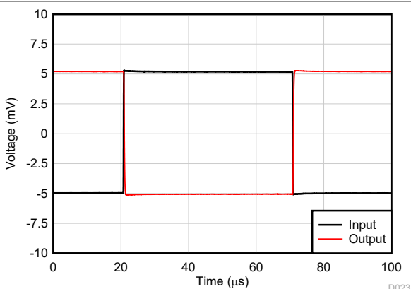
图 5-28. 过载恢复
