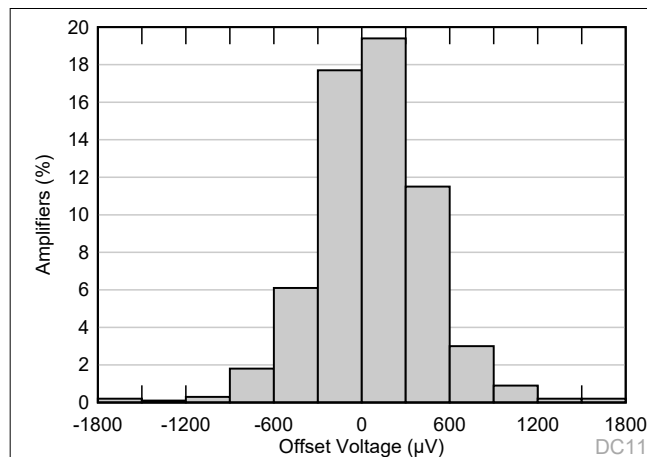
图 5-1. 失调电压生产分配
