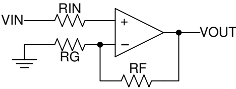
图 8-4. 同相配置的运算放大器原理图
