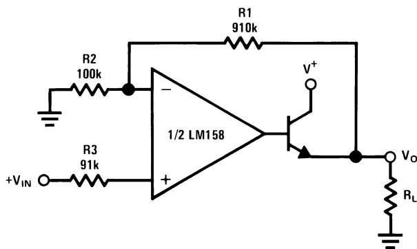
图 8-4. Power Amplifier
