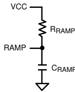
图 6-7. V OUT > 7.5V 时，R RAMP 连接 V CC
