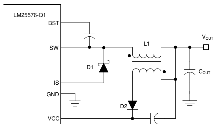
图 7-5. 8V < V_{OUT} < 14V 时来自 V_{OUT} 的 V_{CC} 偏置
