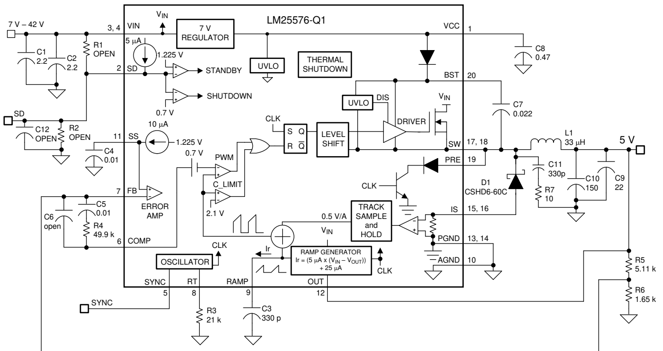
图 6-1. 功能方框图
