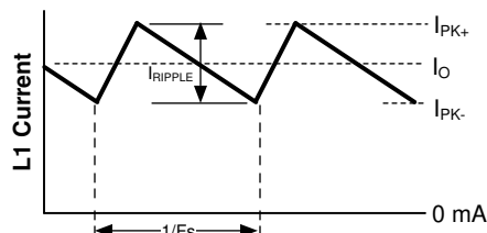
图 7-1. 电感器电流波形
