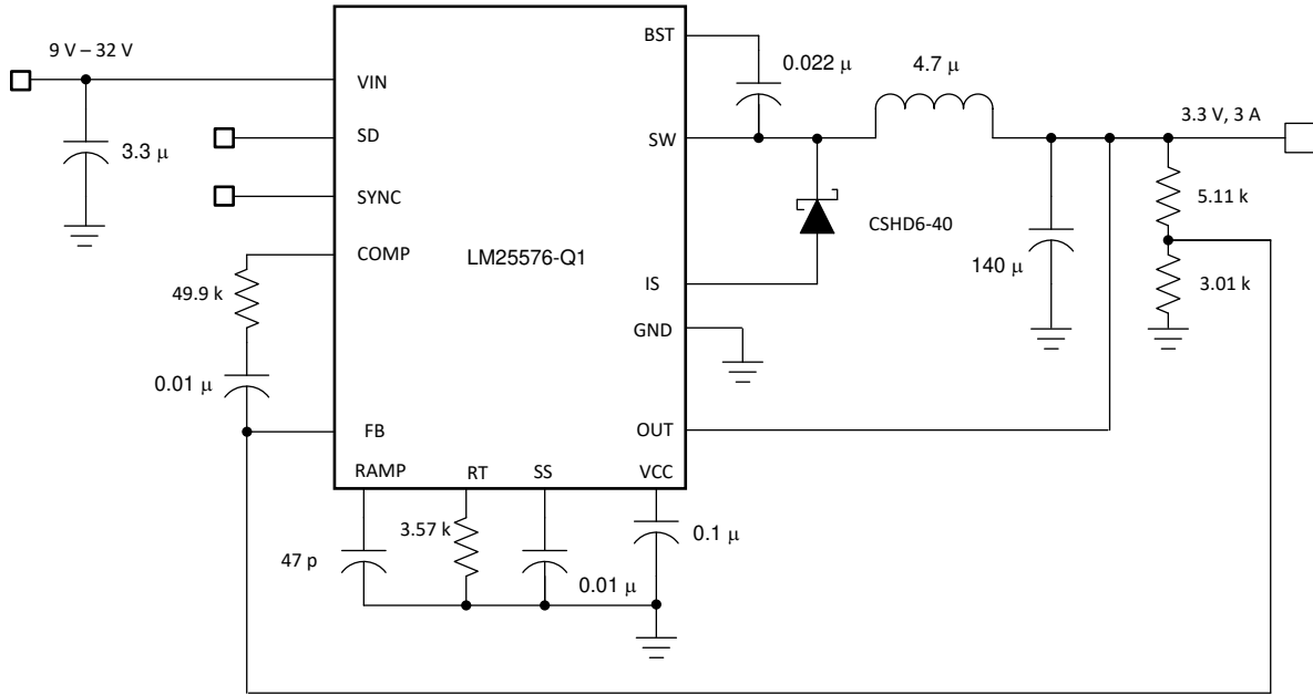
图 7-7. 3.3V、3A、1MHz 原理图
