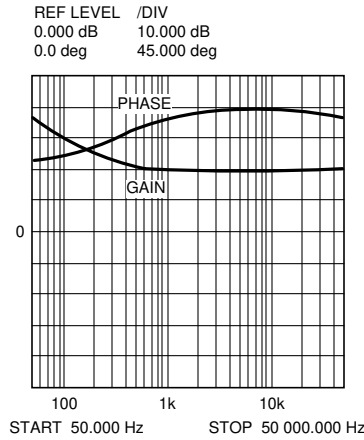
图 7-3. 误差放大器增益与相位
