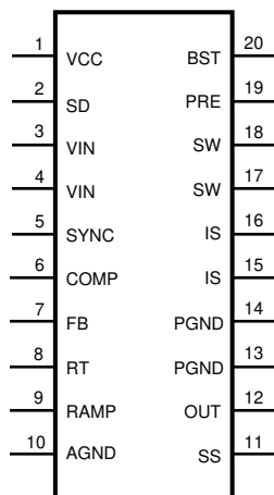
图 4-1. LM25576-Q1 PWP 20-HTSSOP ( 顶视图 )
