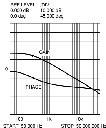
图 7-2. 调制器的增益和相位， R_{\text{LOAD}} = 50\text{ohms} 且 C_{\text{OUT}} = 177\mu\text{F}
