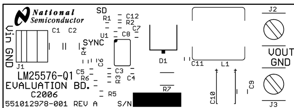
图 7-11. 丝印
