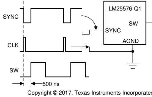
图 6-3. 与外部时钟同步
