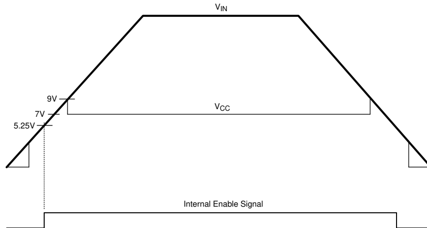
图 6-2. V_{IN} 和 V_{CC} 时序
