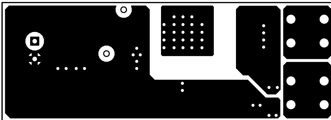
图 7-10. 焊接侧
