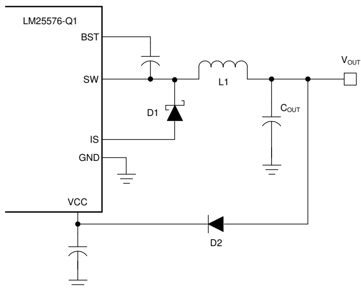
图 7-5. 8V < V_{OUT} < 14V 时来自 V_{OUT} 的 V_{CC} 偏置
