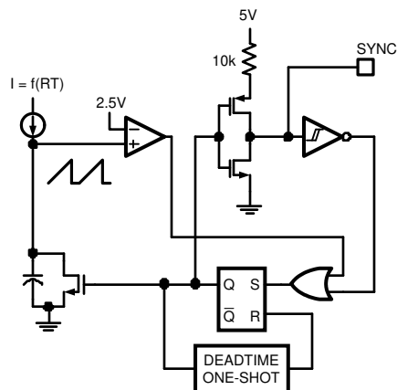
图 6-5. 简化的振荡器方框图及同步 I/O 电路
