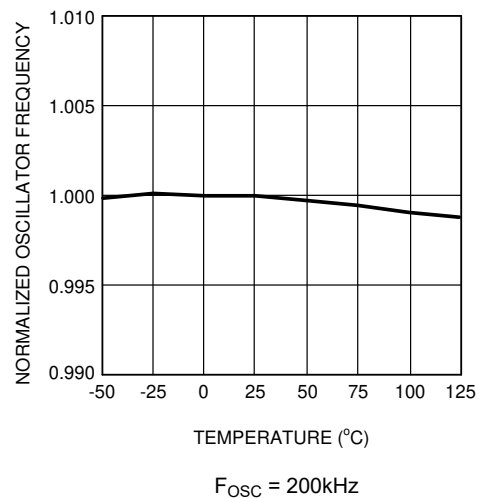
图 5-2. 振荡器频率与温度间的关系
