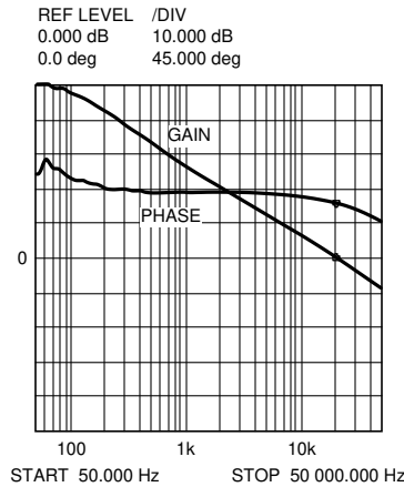
图 7-4. 总体环路增益与相位
