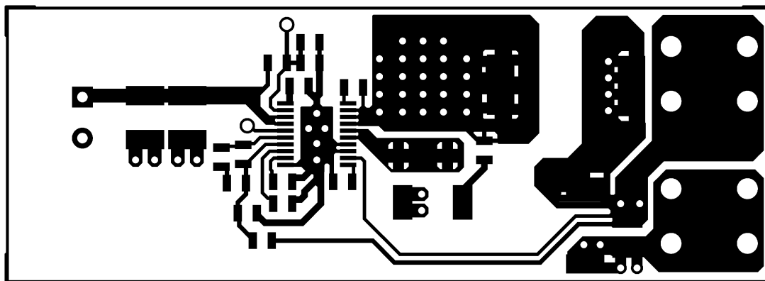
图 7-9. 组件侧
