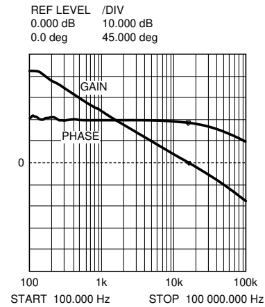
图 7-8. 总体环路增益与相位
