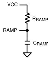
图 6-3. V_{OUT} > 7.5\text{V} 时， R_{RAMP} 连接 V_{CC}
