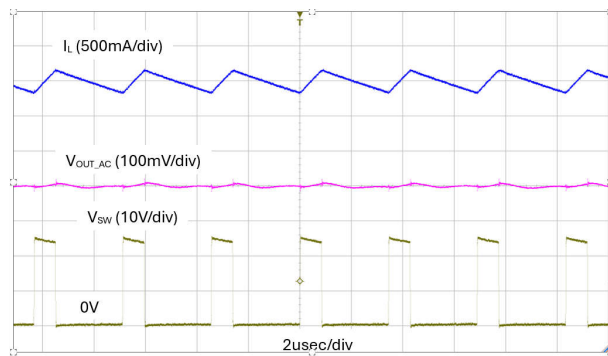
图 7-9. 稳态波形
