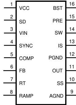
图 4-1. PWP 16 脚 HTSSOP ( 顶视图 )
