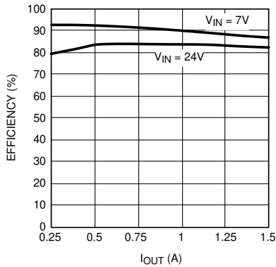
图 7-7. 电路板效率与 I_{OUT} 和 V_{IN} 间的关系
