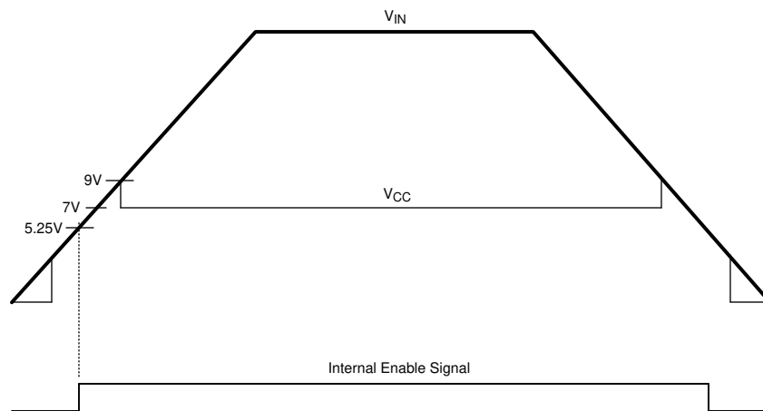
图 6-1. Vin 和 Vcc 时序要求
