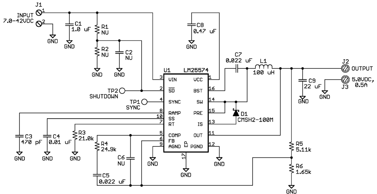
图 7-1. LM25574 Reference Schematic
