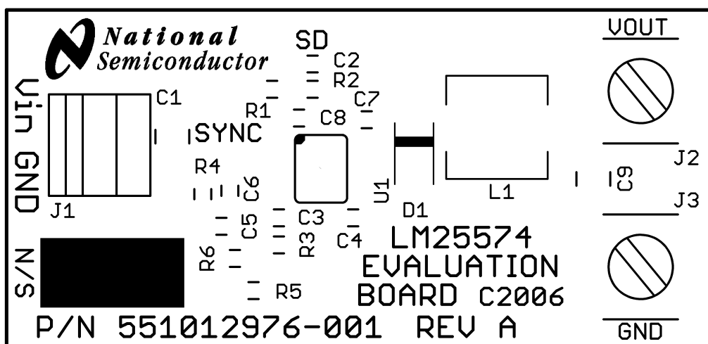
图 7-14. Silkscreen
