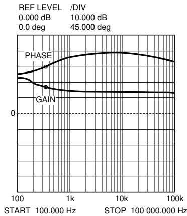
图 7-4. Error Amplifier Gain and Phase
