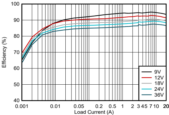
LM25192-Q1 效率, Vout = 6V
