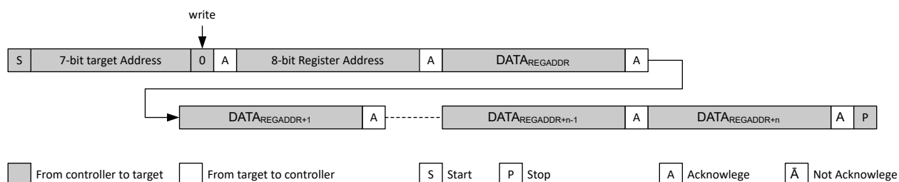
图 8-7. 在定义的寄存器地址开始进行顺序写入
