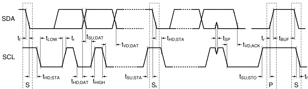
图 8-2. I 2 C 数据传输时序
