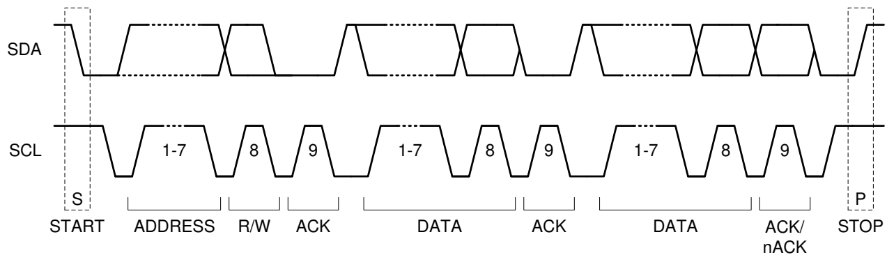
图 8-1. I 2 C 启动/停止/确认协议
