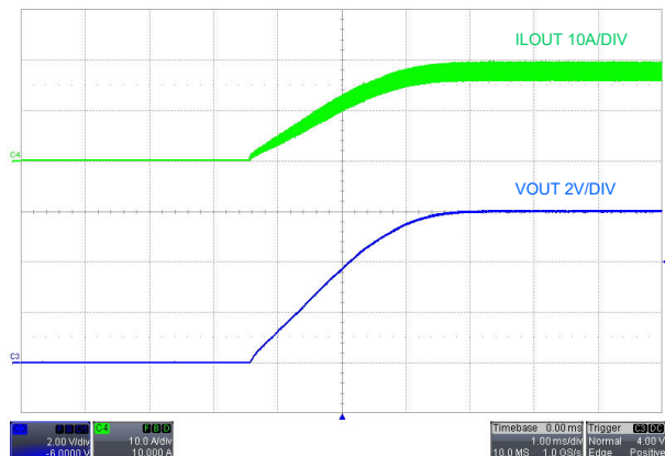
图 10-5. 启动, EN 开启, V_{\text{SUPPLY}} = 12\text{V} , I_{\text{LOAD}} = 18\text{A} 电阻负载
