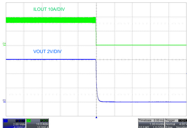
图 10-6. 关断, EN 关闭, V_{\text{SUPPLY}} = 12\text{V} , I_{\text{LOAD}} = 18\text{A} 电阻负载
