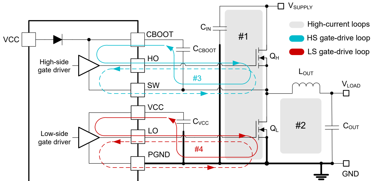
图 10-11. 具有功率级和栅极驱动电路开关环路的直流/直流稳压器接地系统
