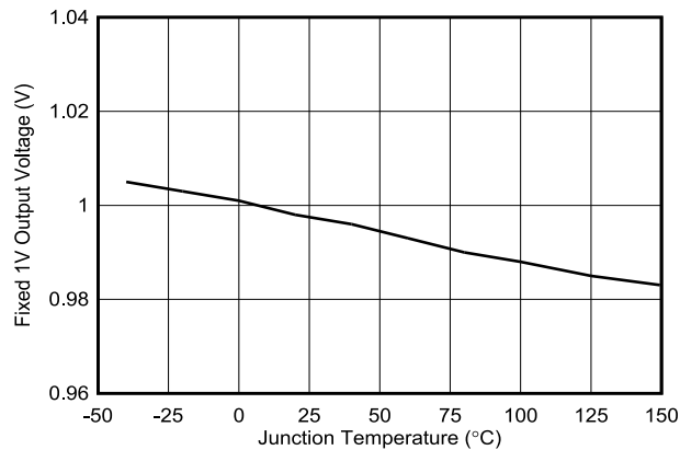
图 6-5. 固定输出电压与温度间的关系, V_{OUT} = 1V
