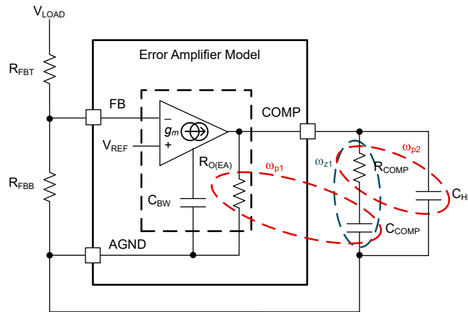
图 10-3. 误差放大器和补偿网络
