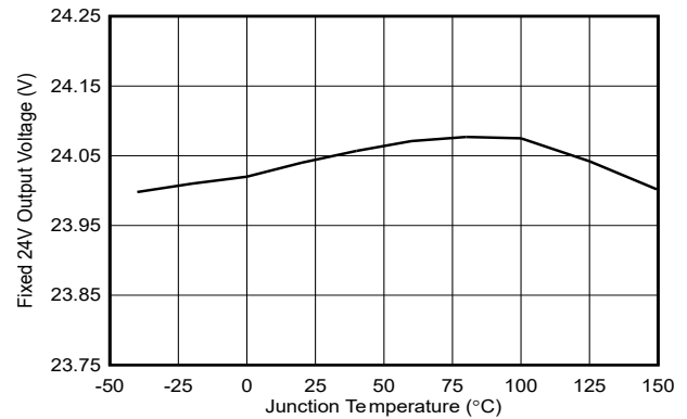
图 6-8. 固定输出电压与温度间的关系, V_{\text{OUT}} = 24\text{V}
