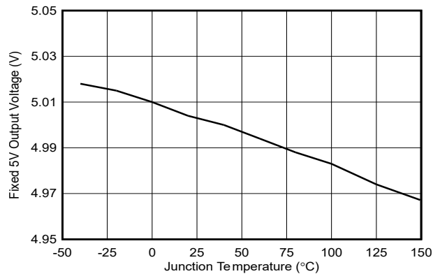
图 6-7. 固定输出电压与温度间的关系, V_{\text{OUT}} = 5\text{V}
