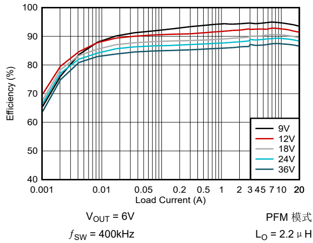
图 6-1. 效率 PFM 模式
