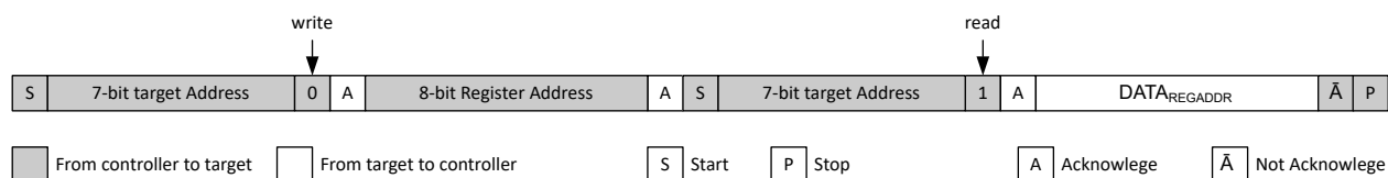
图 8-4. 从定义的寄存器地址进行单次读取
