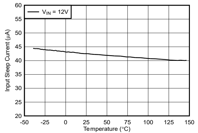
图 6-4. 输入睡眠电流与温度间的关系, V_{OUT} = 5V
