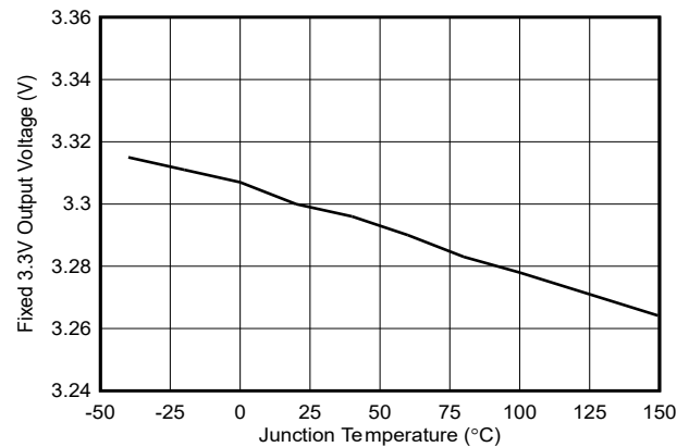
图 6-6. 固定输出电压与温度间的关系, V_{OUT} = 3.3V
