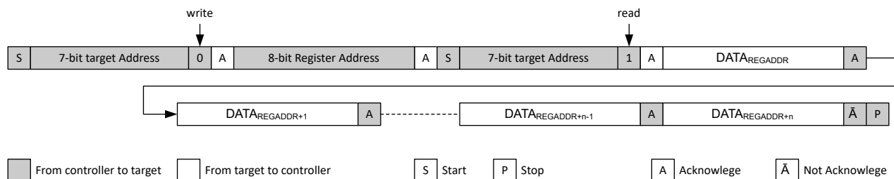
图 8-5. 从定义的寄存器地址开始进行顺序读取
