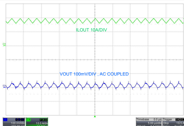
图 10-7. 输出纹波, V_{\text{SUPPLY}} = 12\text{V} , I_{\text{LOAD}} = 18\text{A}
