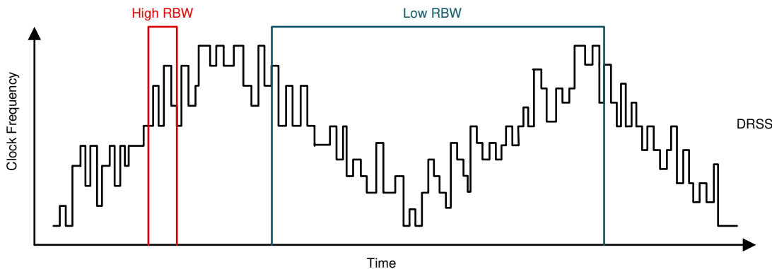
图 7-2. 双随机展频实现
