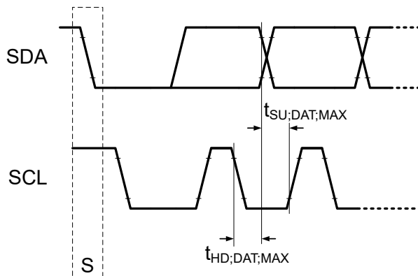
图 8-3. 最长上升和下降时间的 I 2 C 数据传输时序
