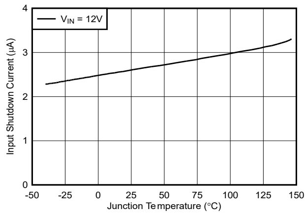
图 6-3. 输入关断电流与温度间的关系
