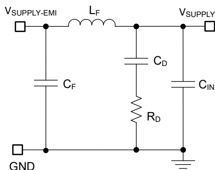
图 10-2. 降压稳压器的无源 \pi 级 EMI 滤波器
