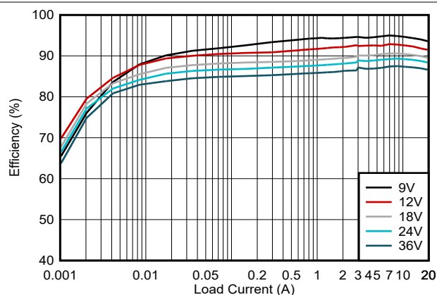
图 10-9. PFM 模式效率, 对数标度
