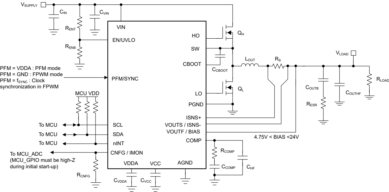
图 10-4. 具有 I 2 C 接口的应用电路
