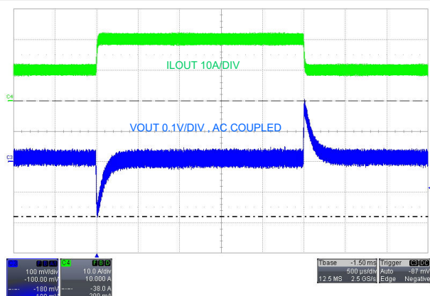
图 10-8. V_{\text{SUPPLY}} = 12\text{V} 、FPWM、从 10A 变为 20A 时的负载瞬态响应
