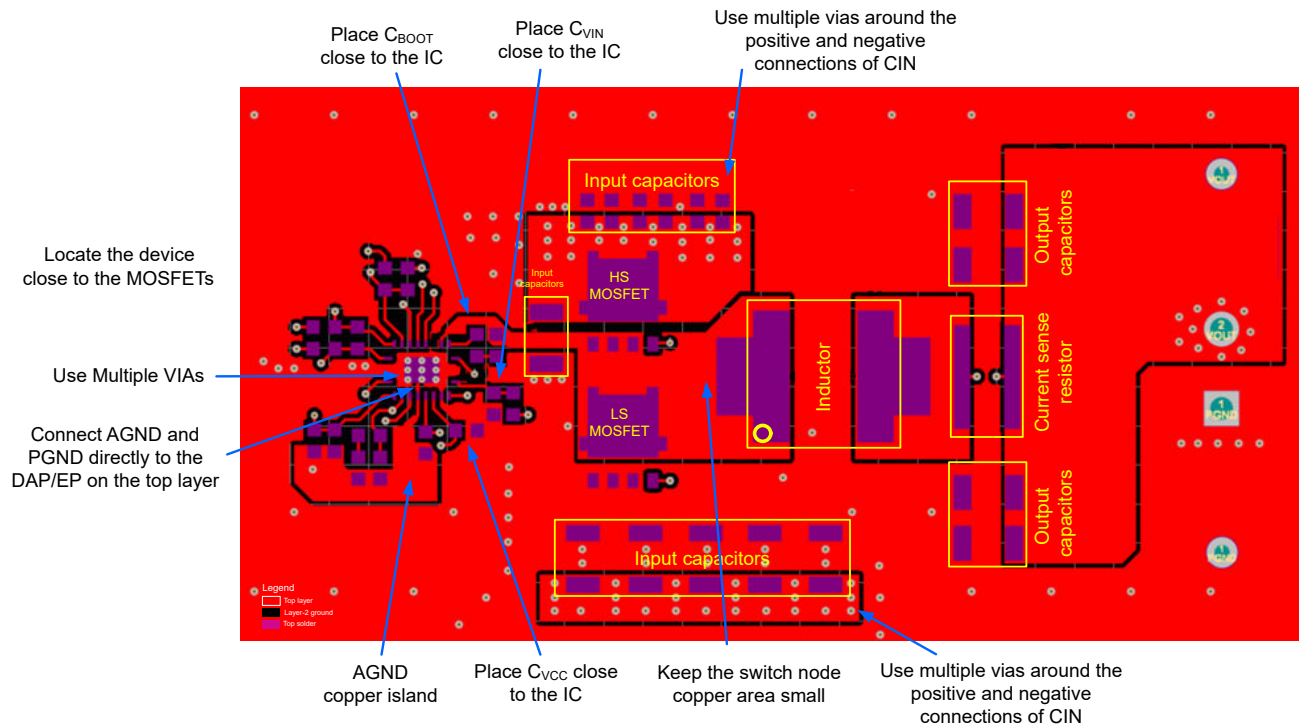
图 10-12. PCB 顶层
