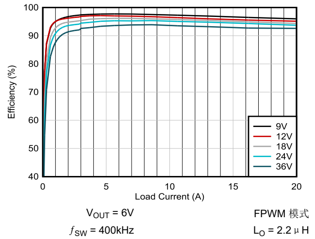
图 6-2. 效率 FPWM 模式
