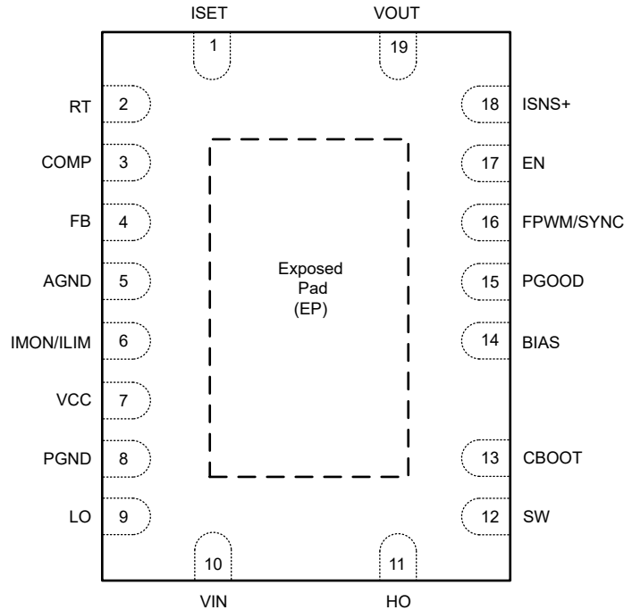
图 4-1. 19 引脚 VQFN RGY 封装（顶视图）
