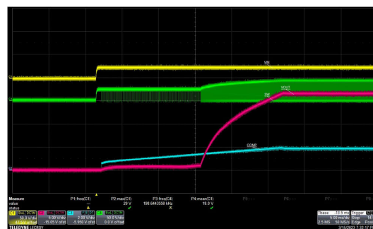
VIN 阶跃至 24V 1A 负载
