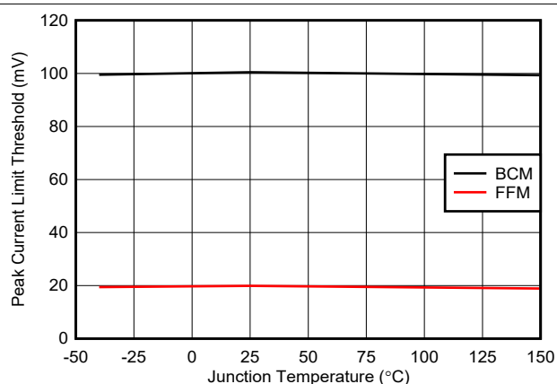
图 6-10. 峰值电流限制阈值与温度间的关系
