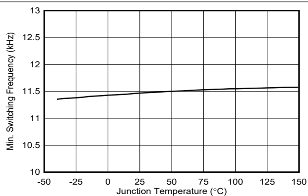
图 6-12. 最小开关频率与温度间的关系
