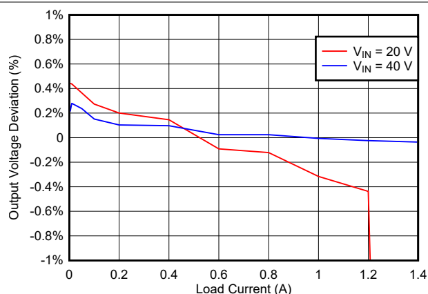
图 8-3. 负载调整率
