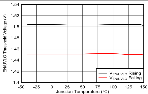
图 6-8. EN/UVLO 阈值电压与温度间的关系
