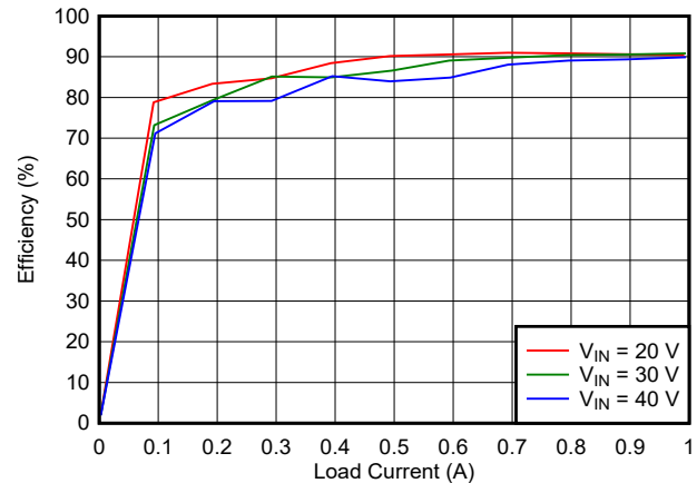
图 3-1. 典型效率 (V OUT = 16.4 V)
