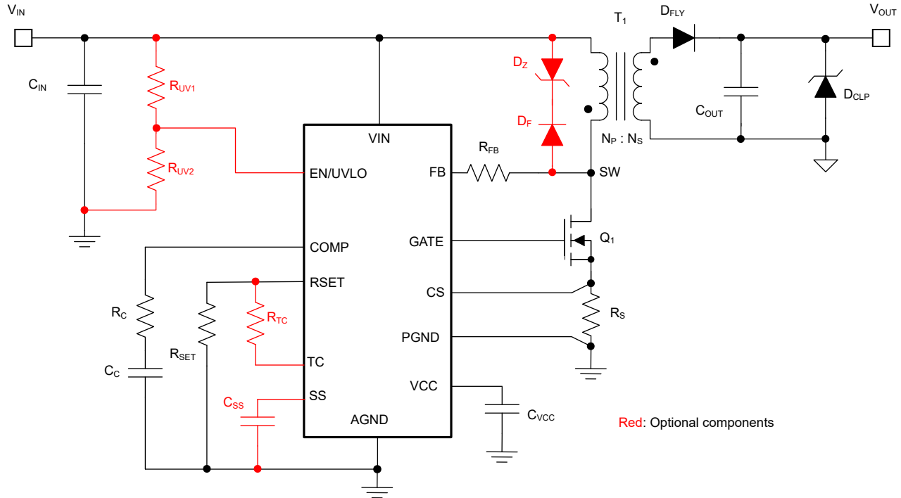
图 7-1. LM25185 反激式转换器原理图 ( 可选元件以红色显示 )
