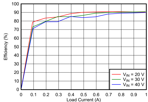
图 3-1. 典型效率 ( V_{OUT} = 16.4\text{ V} )
