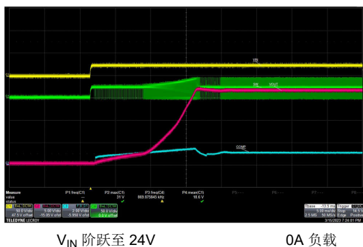
图 8-4. 空载时的启动特性
