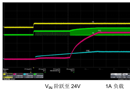
图 8-5. 满载时的启动特性
