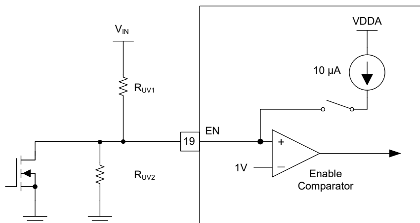
图 8-2. 可编程输入电压 UVLO 导通
