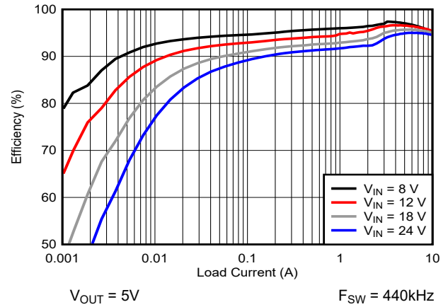
图 7-2. 效率与负载间的关系，对数标度
