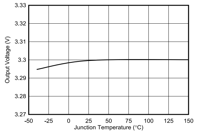
图 7-6. 3.3V 固定输出电压与温度间的关系
