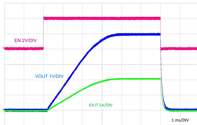
图 9-25. 使能端开启和关闭特性
