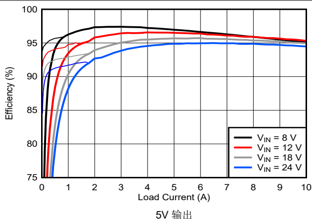
图 9-18. 效率与 I_{OUT} 之间的关系
