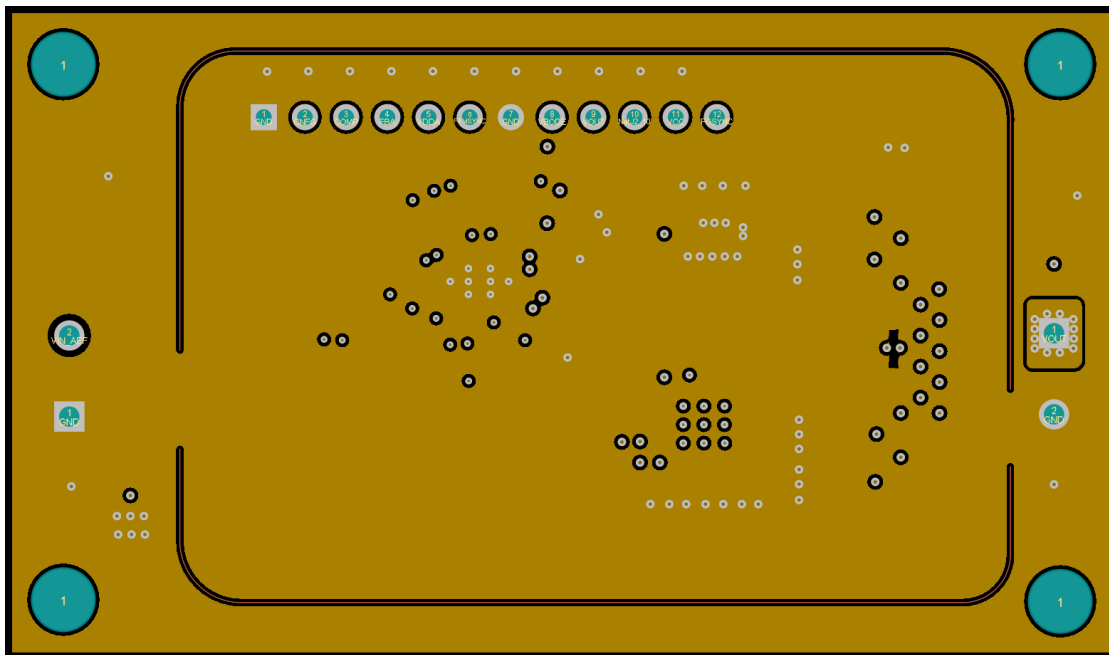
图 9-37. 电源元件正下方的第 2 层完整接地平面
