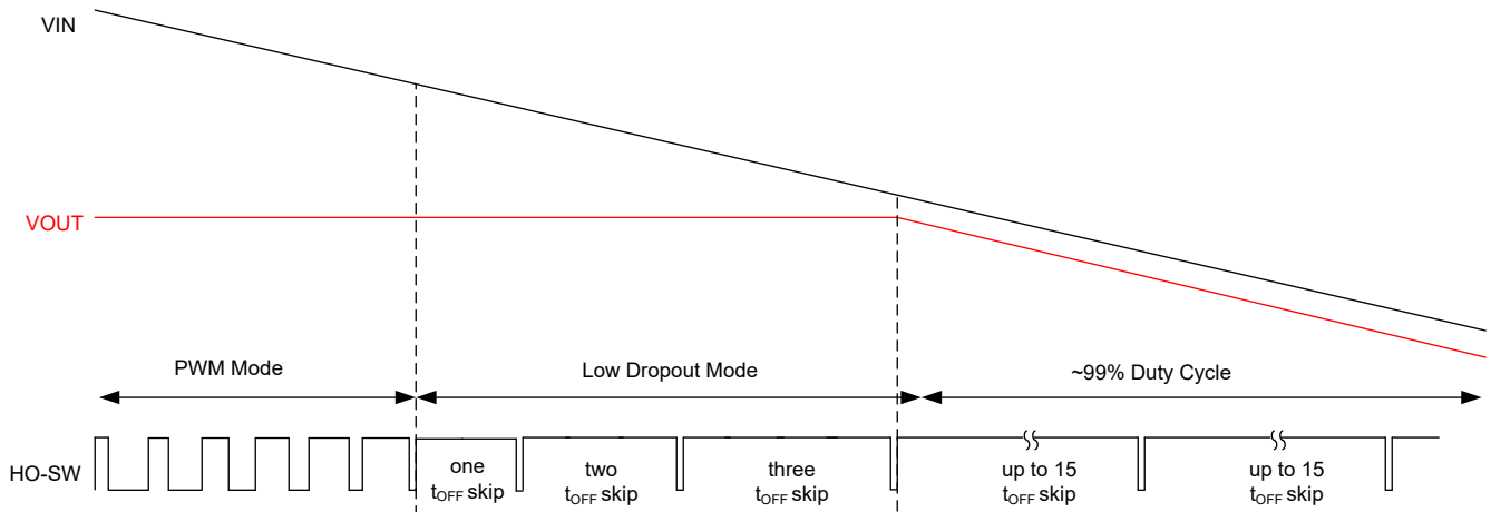
图 8-1. 压降模式运行
