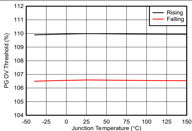
图 7-9. PG OV 阈值与温度间的关系
