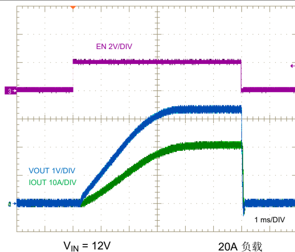
图 9-32. 使能端开启和关闭特性
