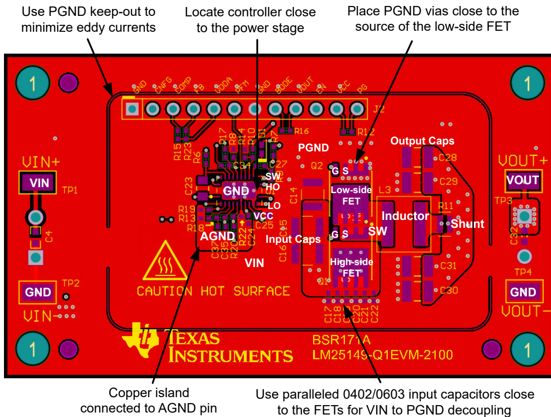
图 9-36. PCB 顶层 - 高密度单面设计
