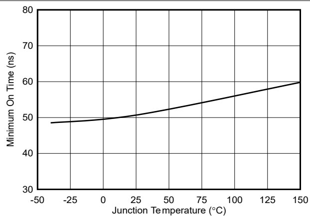
图 7-19. 最短导通时间 (HO) 与温度间的关系
