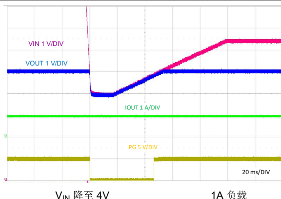
图 9-23. V_{IN} = 4V 时的线路瞬态响应
