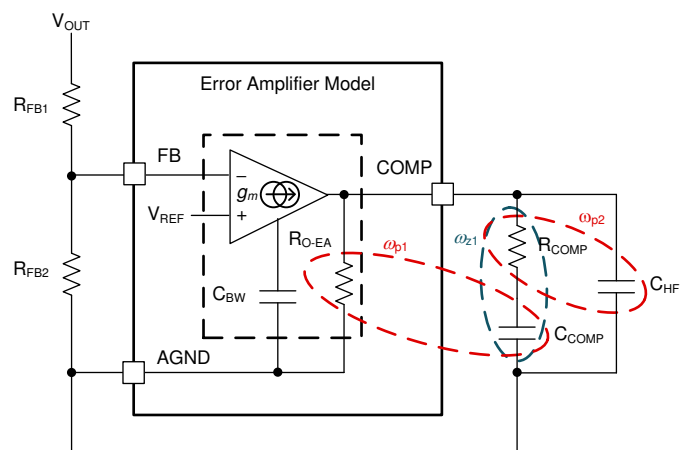
图 9-3. 误差放大器和补偿网络
