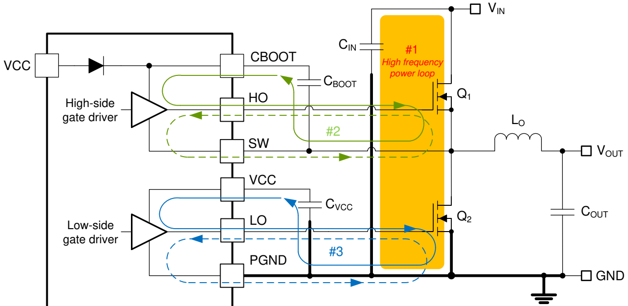
图 9-35. 具有功率级和栅极驱动电路开关环路的直流/直流稳压器接地系统
