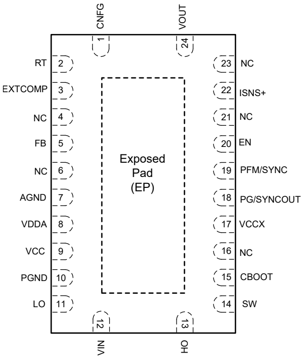
图 6-2. 具有可湿性侧面的 24 引脚 VQFN RGY 封装，LM25148BQRGYRQ1（顶视图）
