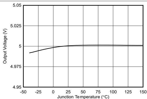
图 7-7. 5V 固定输出电压与温度间的关系
