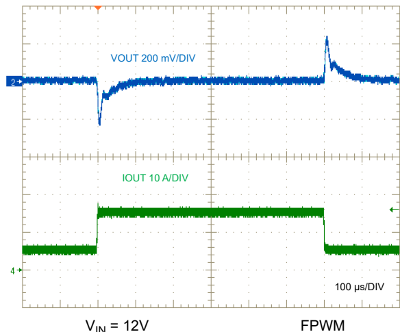
图 9-33. 负载瞬态，5A 至 15A
