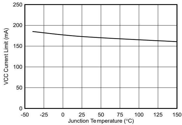
图 7-13. VCC 电流限值与温度间的关系
