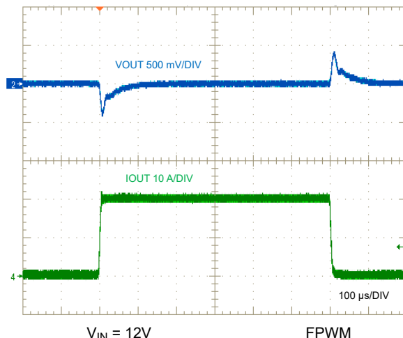
图 9-34. 负载瞬态，0A 至 20A
