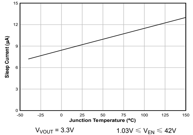
图 7-4. Sleep1 电流与温度间的关系
