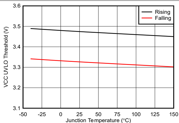
图 7-12. VCC UVLO 阈值与温度间的关系
