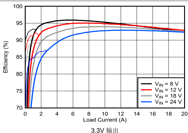
图 9-29. 效率与 I_{OUT} 之间的关系
