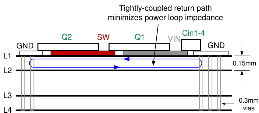
图 9-38. 具有低 L1-L2 层内间距的 PCB 堆叠原理图 1
