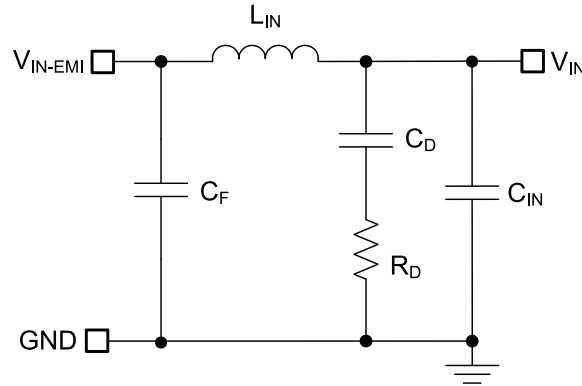
图 9-2. 降压稳压器的无源 \pi 级 EMI 滤波器
