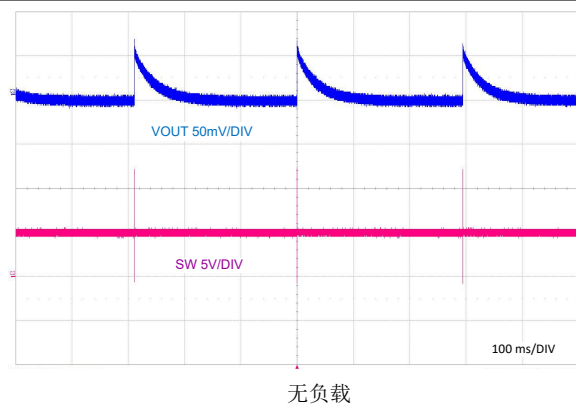
图 9-21. PFM 开关
