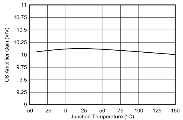
图 7-18. 电流检测 (CS) 放大器增益与温度间的关系
