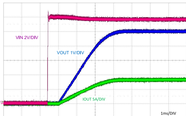
图 9-11. 启动特性
