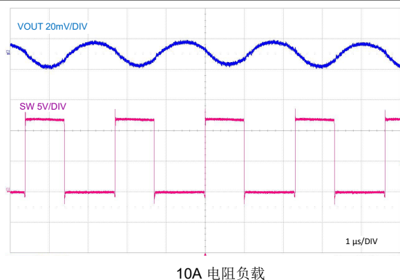
图 9-20. 满负载开关
