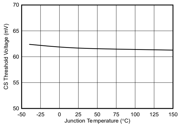
图 7-17. 电流检测 (CS) 阈值与温度间的关系
