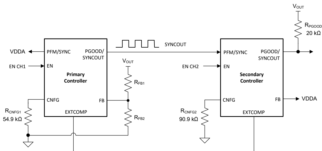
图 8-7. 单输出双相操作的配置原理图
