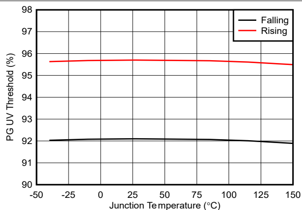
图 7-10. PG UV 阈值与温度间的关系
