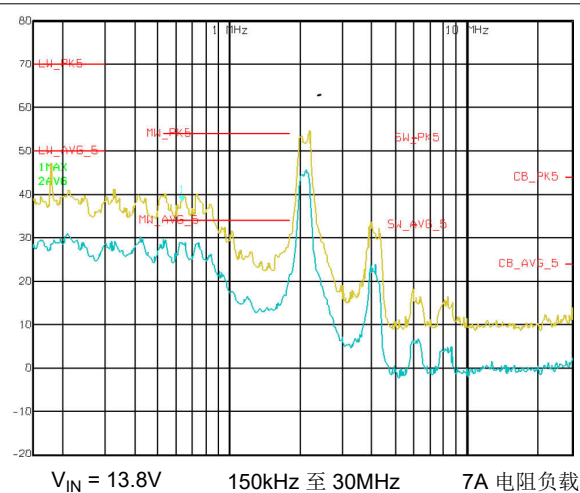
图 9-16. CISPR 25 5 类传导 EMI
