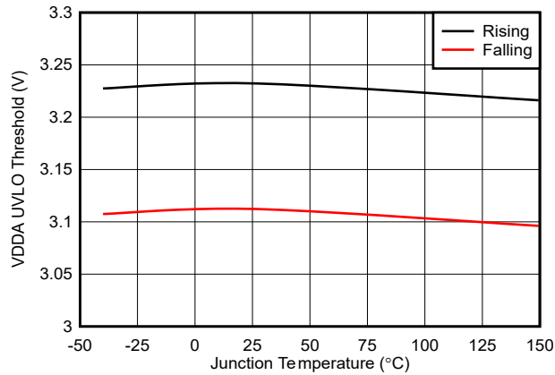
图 7-15. VDDA UVLO 阈值与温度间的关系
