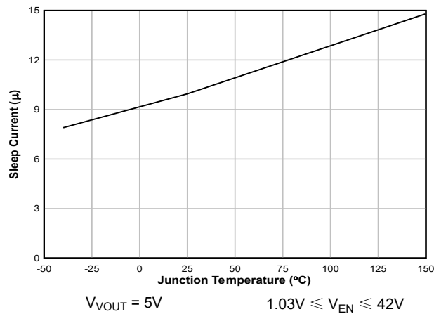
图 7-5. Sleep2 电流与温度间的关系
