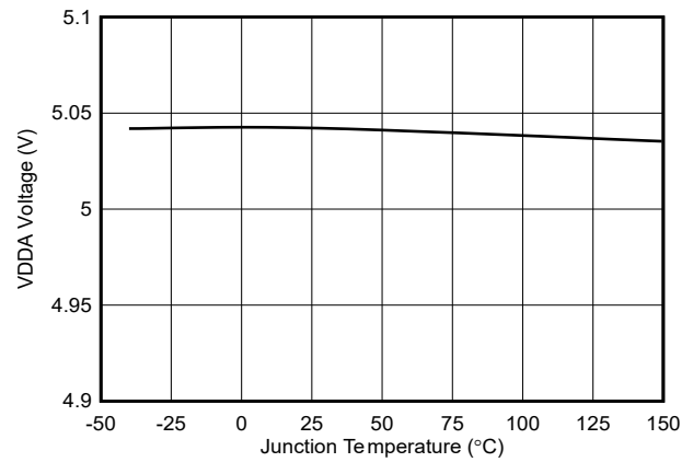
图 7-14. VDDA 稳压电压与温度间的关系
