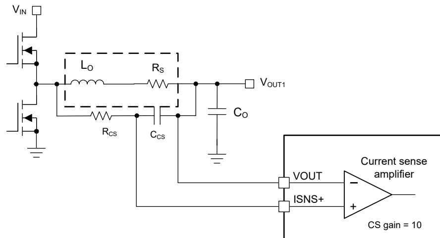
图 8-5. 电感器 DCR 电流检测实现方案
