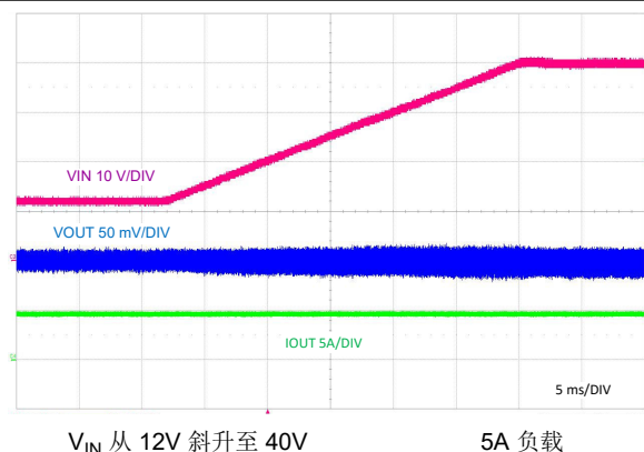
图 9-22. V_{IN} = 40V 时的线路瞬态响应
