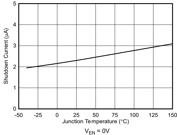
图 7-3. 关断电流与温度间的关系
