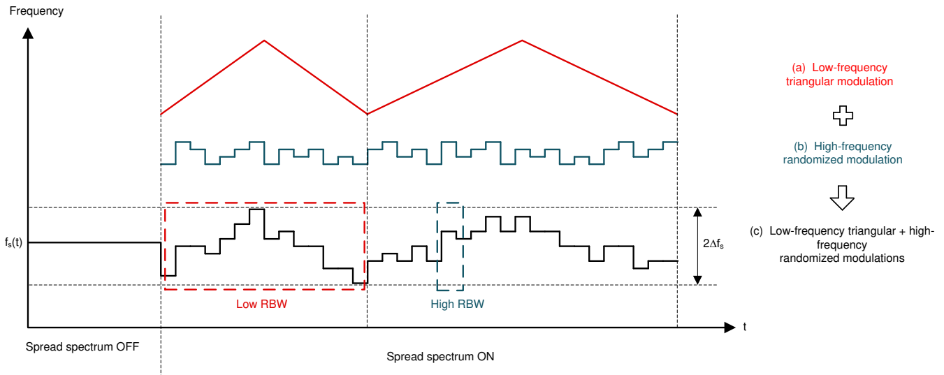
图 8-3. 双随机展频实现
