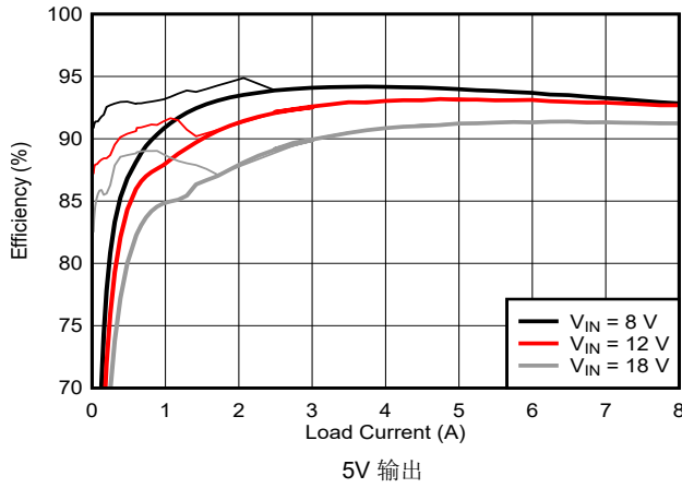
图 9-5. 效率与 I_{OUT} 之间的关系
