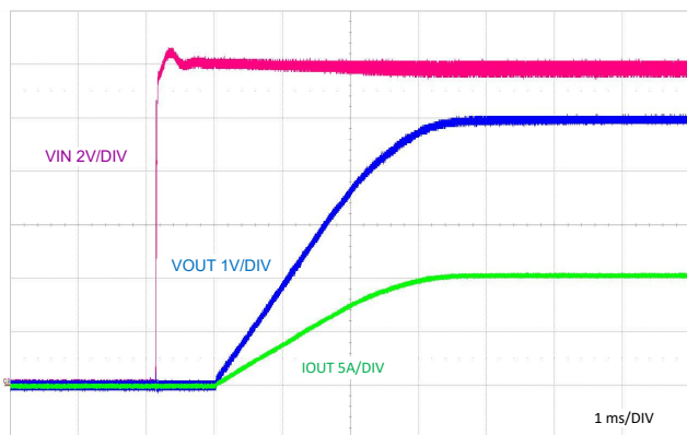
图 9-24. 启动特性
