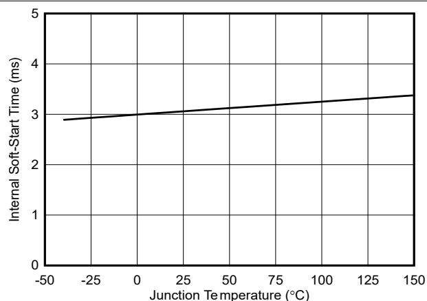
图 7-20. 软启动时间与温度间的关系
