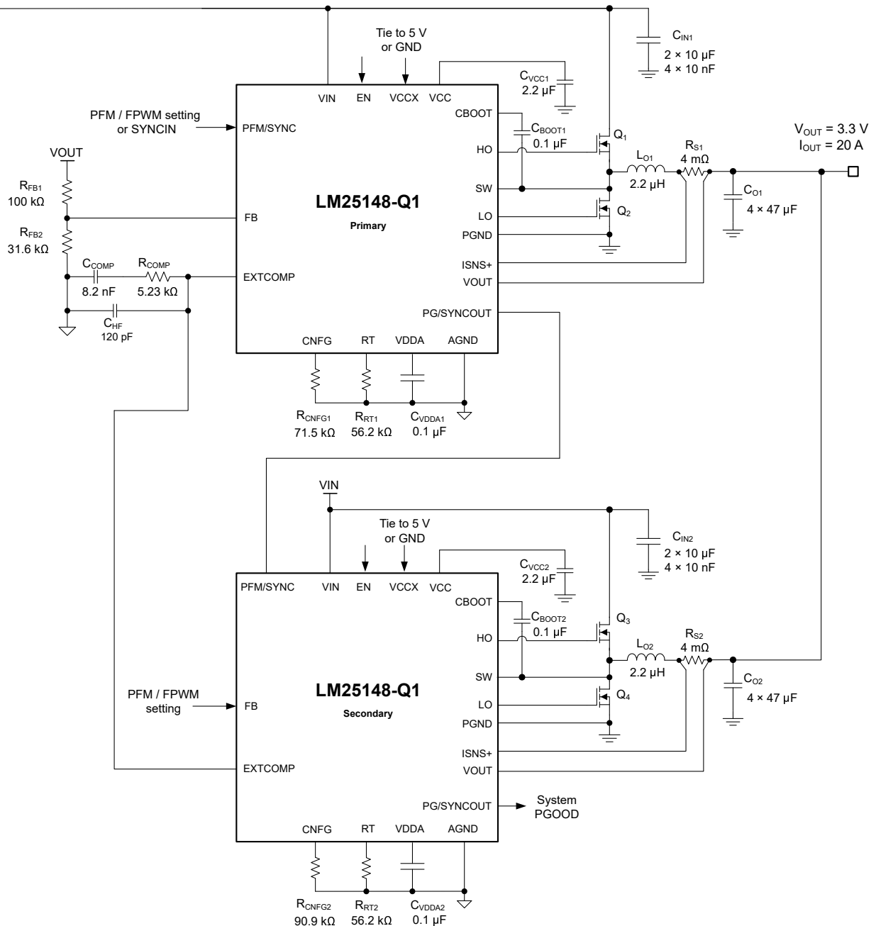
图 9-28. 采用两个 LM25148-Q1 降压稳压器且开关频率为 400kHz 的应用电路 3
