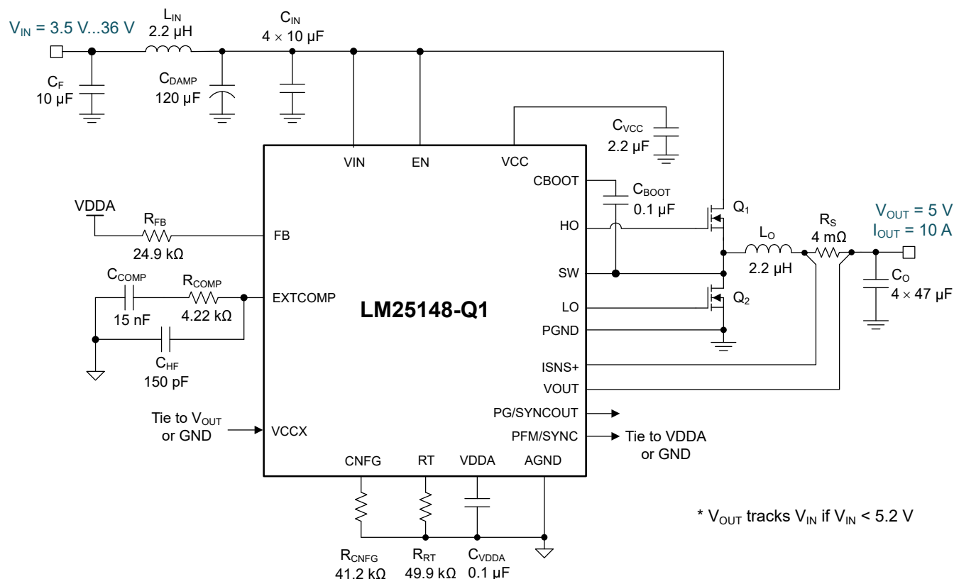
图 9-17. 采用 LM25148-Q1 降压稳压器且开关频率为 440kHz 的应用电路 2
