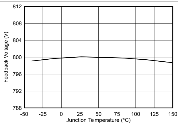
图 7-8. 反馈电压与温度之间的关系
