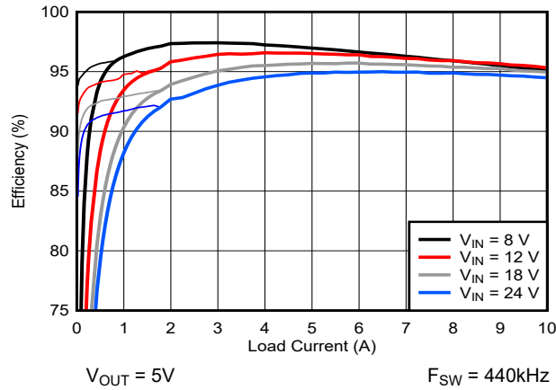
图 7-1. 效率与负载间的关系
