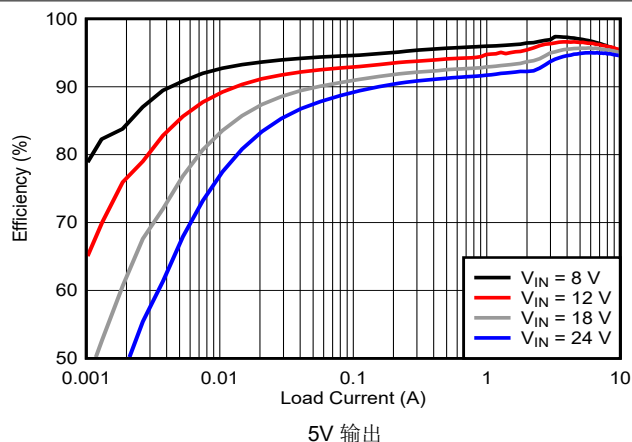
图 9-19. 效率与 I_{OUT} 之间的关系，对数标度
