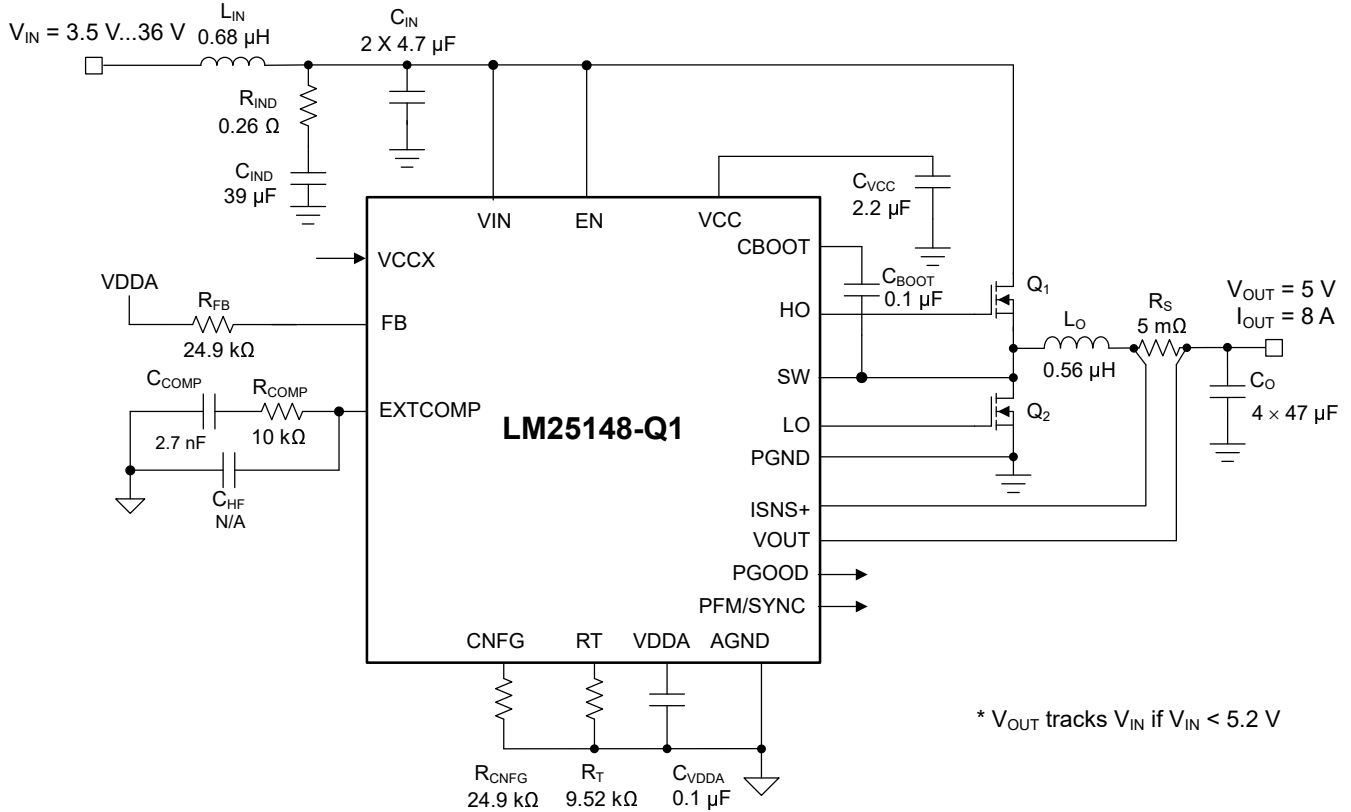
图 9-4. 采用 LM25148-Q1 降压稳压器且开关频率为 2.1MHz 时的应用电路 1
