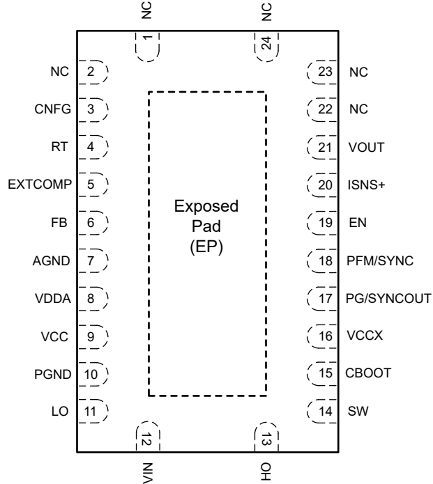
图 6-1. 具有可湿性侧面的 24 引脚 VQFN RGY 封装，LM25148QRGYRQ1（顶视图）
