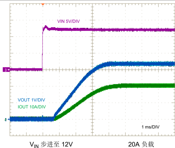
图 9-31. V_{IN} 启动特性
