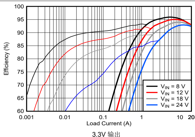
图 9-30. 效率与 I_{OUT} 之间的关系，对数标度
