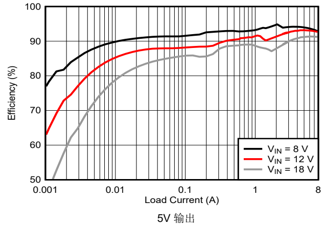
图 9-6. 效率与 I_{OUT} 之间的关系，对数标度
