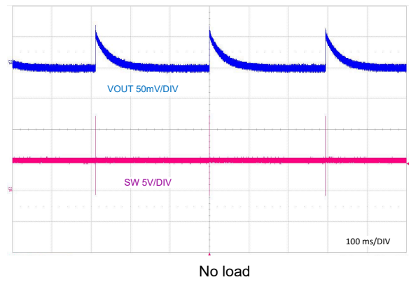
图 9-21. PFM Switching
