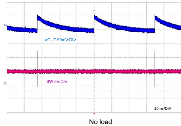
图 9-8. PFM Switching
