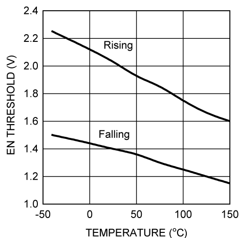
图 5-8. EN Input Threshold vs Temperature
