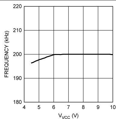
图 6-6. Frequency vs V_{CC}
