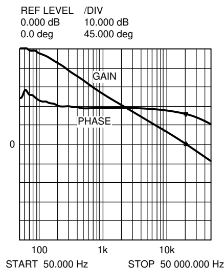
图 7-6. 总体环路增益与相位
