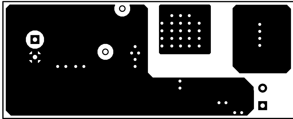
图 7-9. 焊接侧
