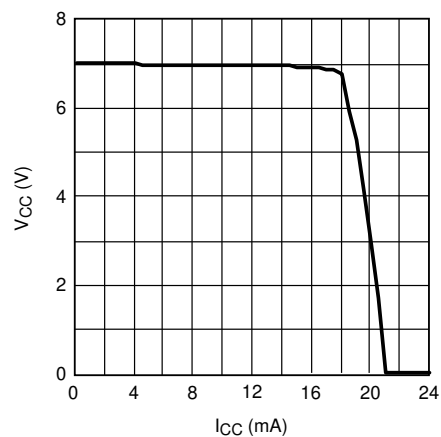
图 5-4. V_{CC} 与 I_{CC} 间的关系 V_{IN} = 12\text{V}
