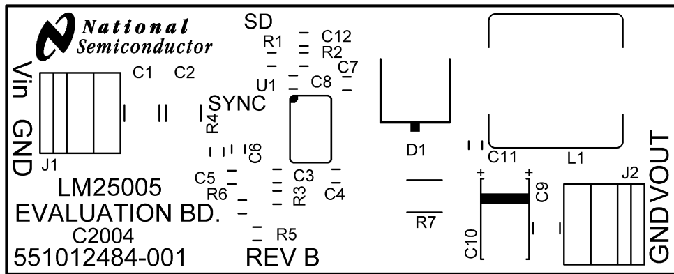
图 7-10. 丝印
