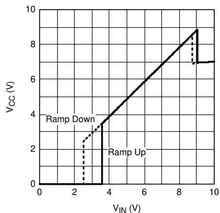
图 5-5. V_{CC} 与 V_{IN} 间的关系 R_L = 7\text{k}\Omega
