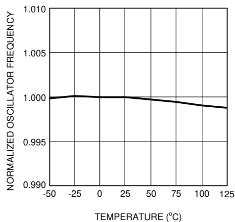
图 5-2. 振荡器频率与温度间的关系 F_{OSC} = 200\text{kHz}
