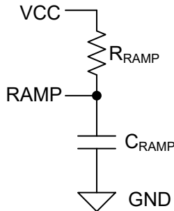
图 6-7. V_{OUT} > 7.5V 时， R_{RAMP} 连接 V_{CC}
