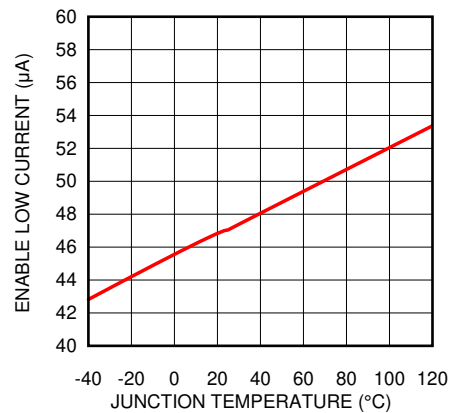
图 6-8. Enable Low Current vs Temperature
