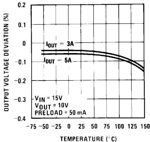
图 4. Load Regulation
