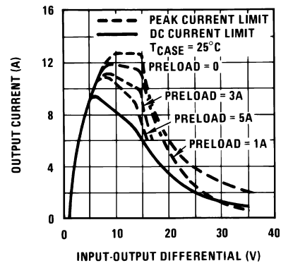
图 5-2. Current Limit
