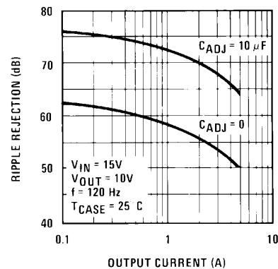
图 5-10. Ripple Rejection
