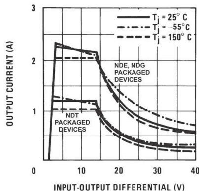
图 7-2. 电流限值
