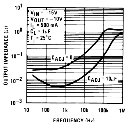
图 5-10. 输出阻抗
