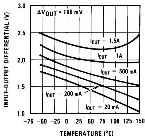
图 7-4. Dropout Voltage
