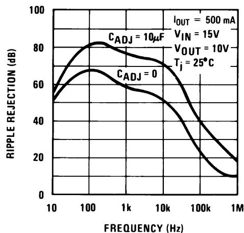
图 7-8. Ripple Rejection
