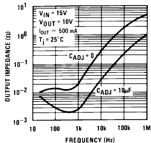
图 7-10. Output Impedance
