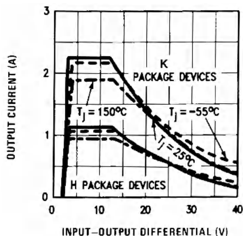
图 7-2. Current Limit
