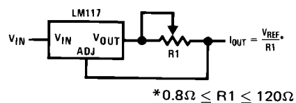
图 9-14. Precision Current Limiter
