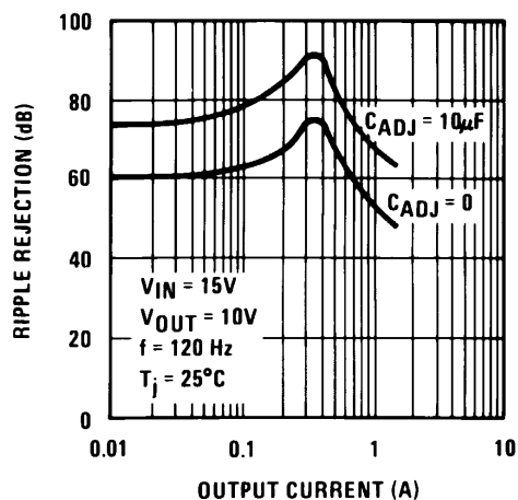
图 7-9. Ripple Rejection
