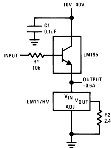
图 9-9. Power Follower
