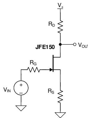
图 9-2. Common-Source Amplifier
