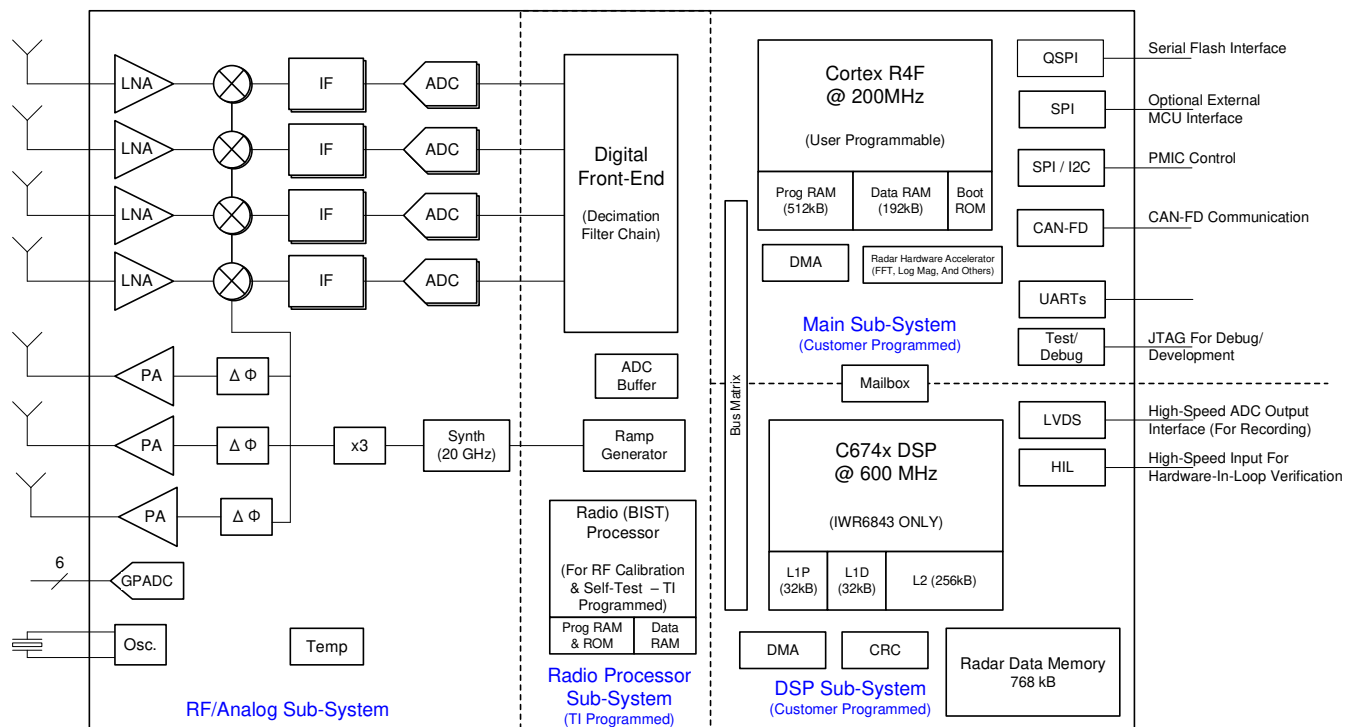
图 4-1. 功能方框图
