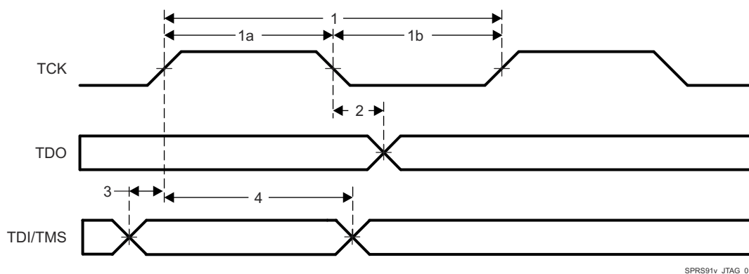
图 6-25. JTAG 时序
