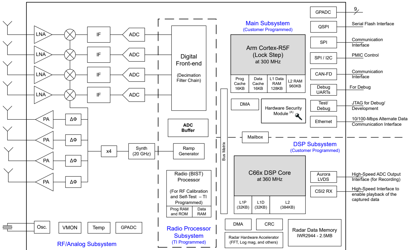
图 3-1. 功能方框图
