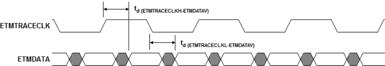
图 6-27. ETMDATA 时序
