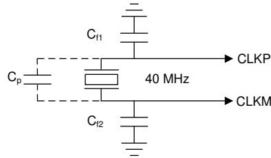
图 6-3. 晶体实现
