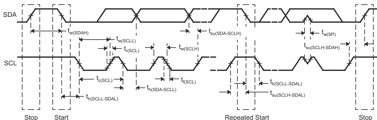
图 6-23. I2C 时序图
