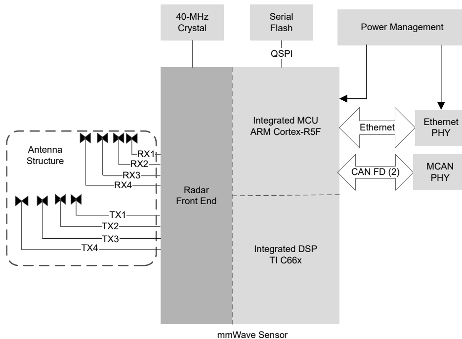
图 9-1. 短距离和中距离雷达
