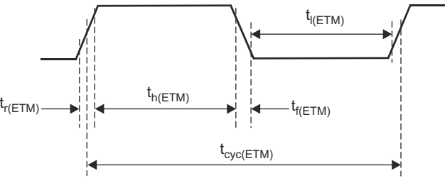
图 6-26. ETMTRACECLKOUT 时序
