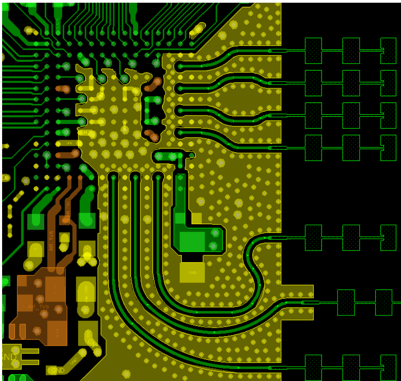
图 11-4. Top Layer Routing Closeup
