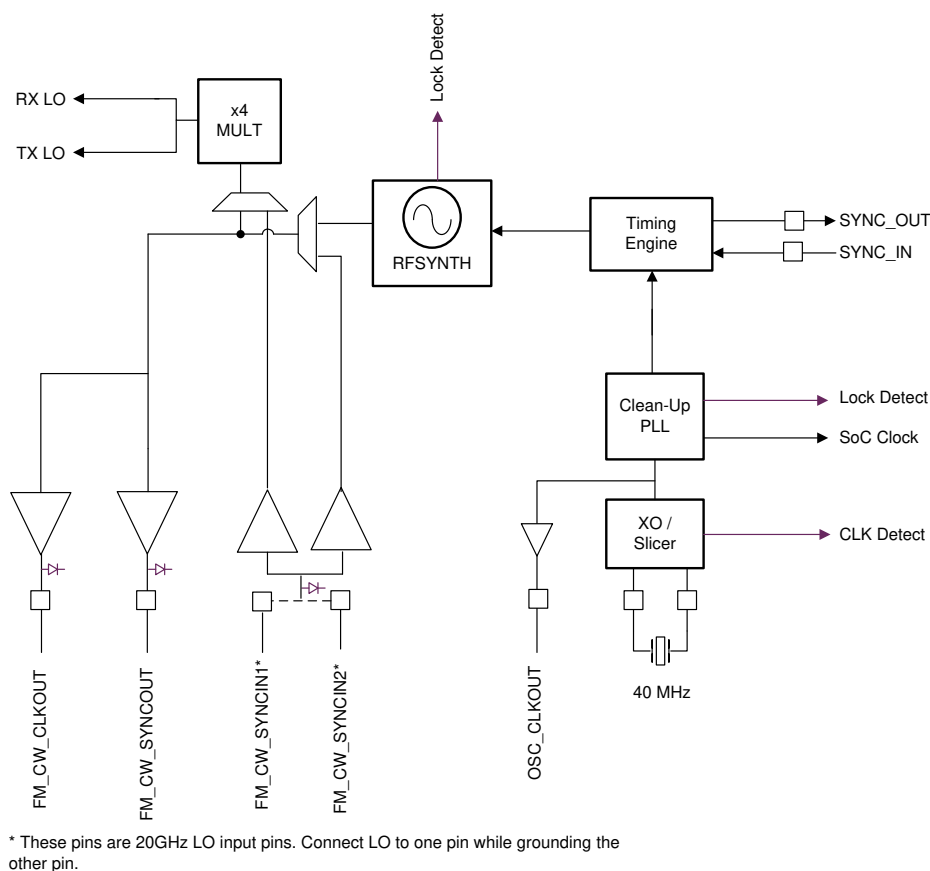
图 9-1. Clock Subsystem
