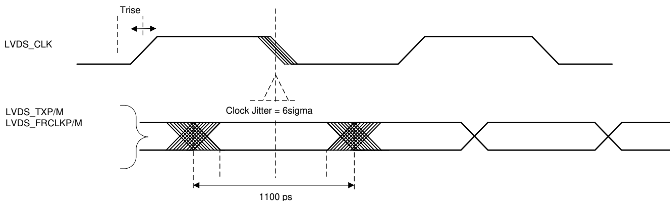
图 8-11. Timing Parameters
