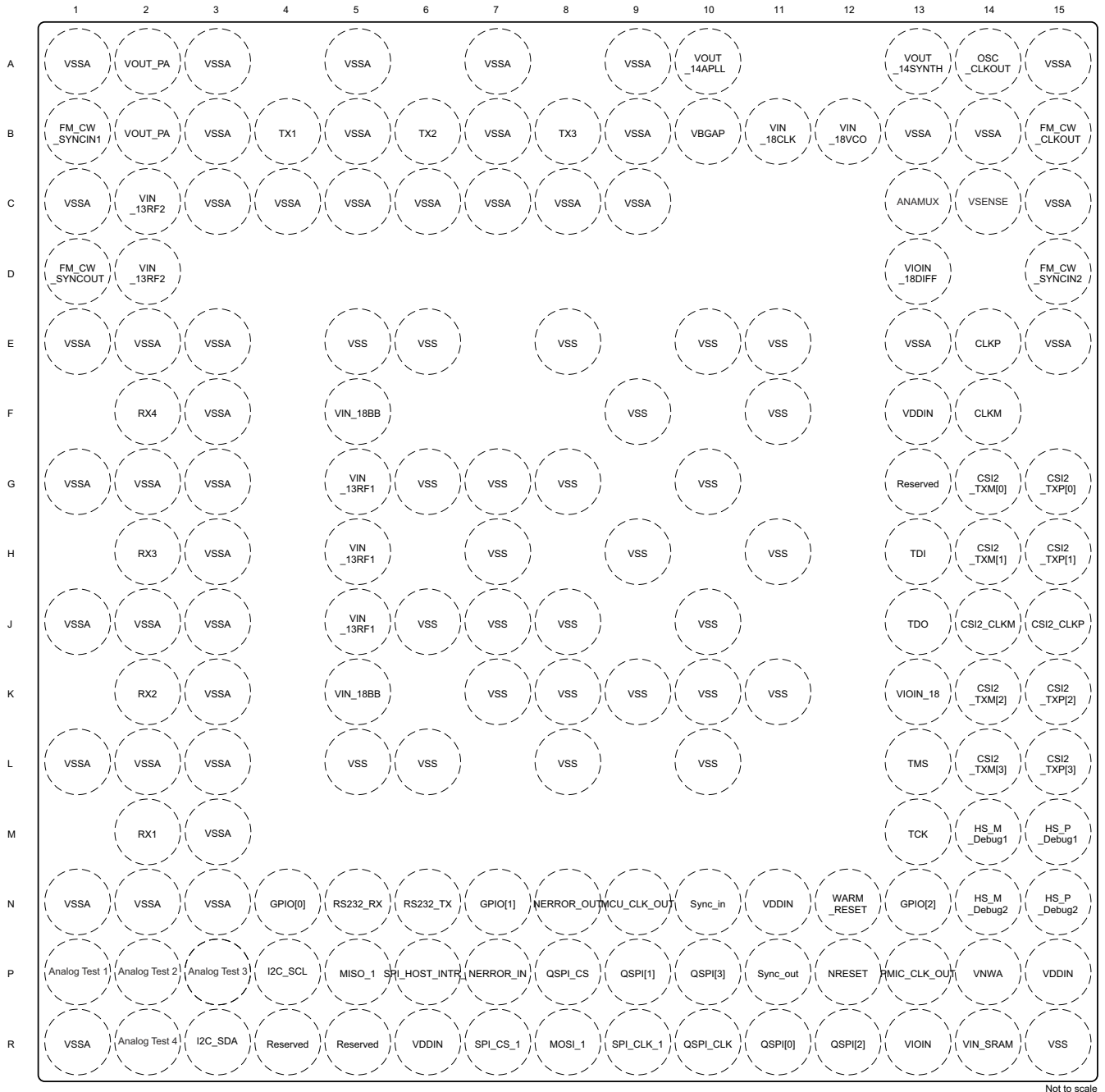
图 7-1. Pin Diagram
