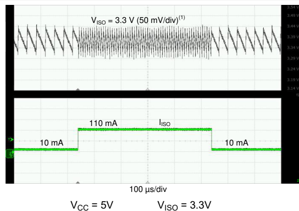
图 7-25. 10 mA 至 110 mA 负载瞬态响应
