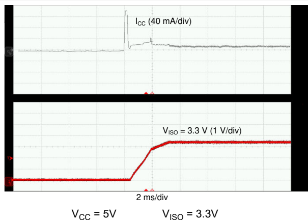
图 7-26. 10 mA 负载条件下的软启动
