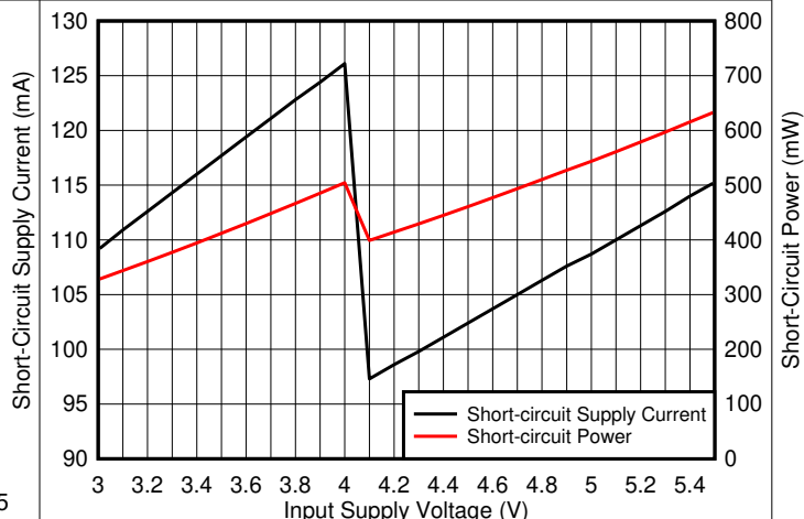
图 7-10. 短路电源电流 ( I_{CC} ) 和功率 ( P ) 与电源电压 ( V_{CC} ) 间的关系
