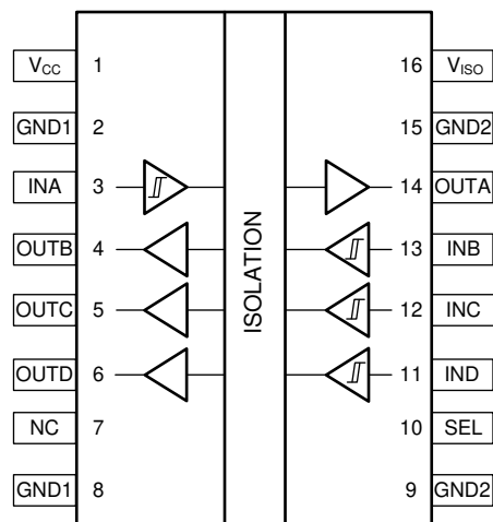
图 6-4. ISOW7843 DWE 封装 16 引脚 SOIC-WB 顶视图
