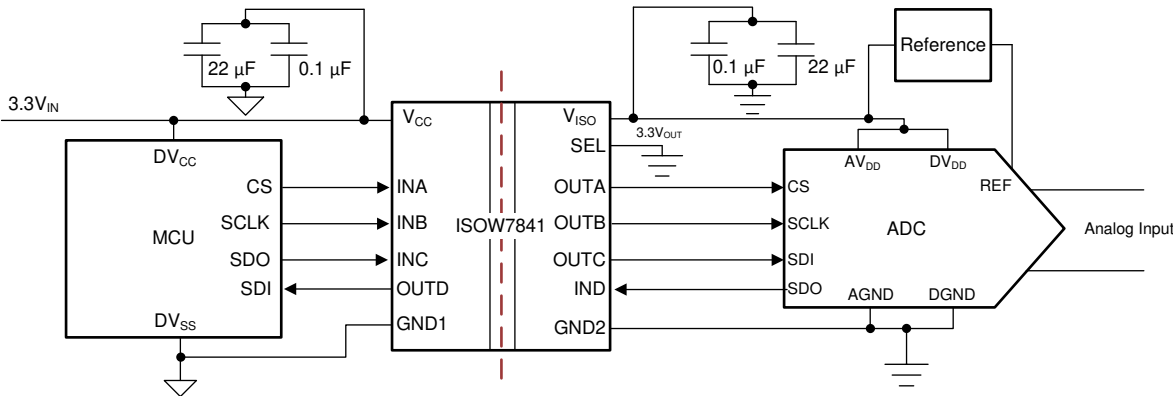
图 10-1. 采用 ISOW7841
