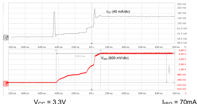
图 10-3. 软启动波形
