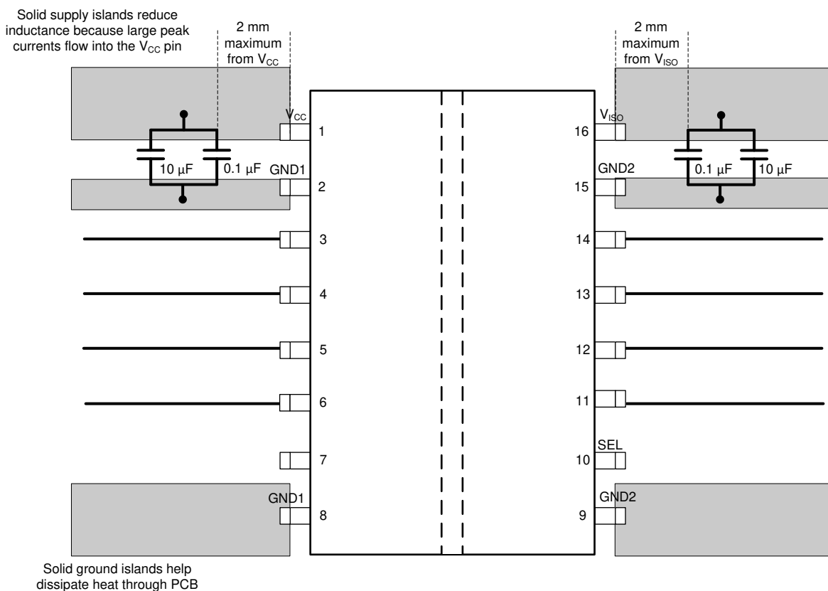
图 12-1. 布局示例
