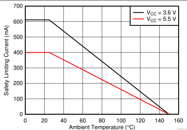
图 7-1. 安全限制电流的热降额曲线 (根据 VDE 标准)
