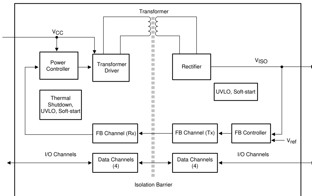
图 9-1. 方框图
