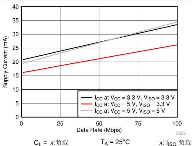
图 7-12. ISOW7840 电源电流与数据速率间的关系
