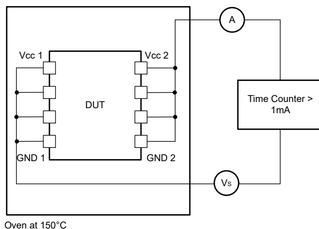
图 8-5. 绝缘寿命测量的测试设置
