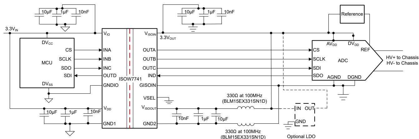
图 8-1. 采用的 ADC 检测应用的隔离式电源与 SPI
