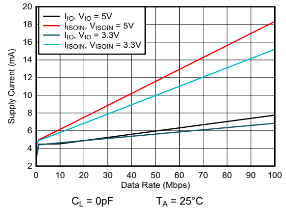
图 5-12. ISOW7741-Q1 通道电源电流与 CL = 0pF 时的数据速率间的关系
