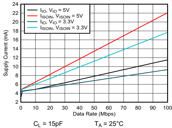
图 5-11. ISOW7741-Q1 通道电源电流与 CL = 15pF 时的数据速率间的关系
