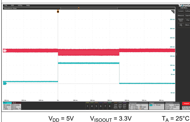
图 5-19. 10mA 至 110mA 负载瞬态响应
