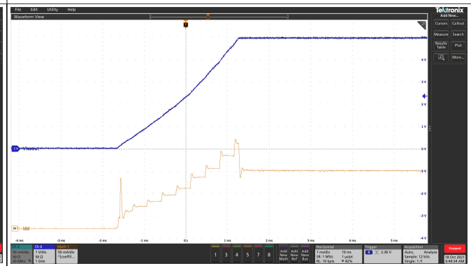
图 5-22. V_{ISOOUT} = 3.3V 时 110mA 负载处的软启动
