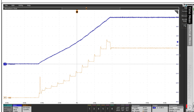
图 5-23. V_{ISOOUT} = 5V 时 10mA 负载处的软启动
