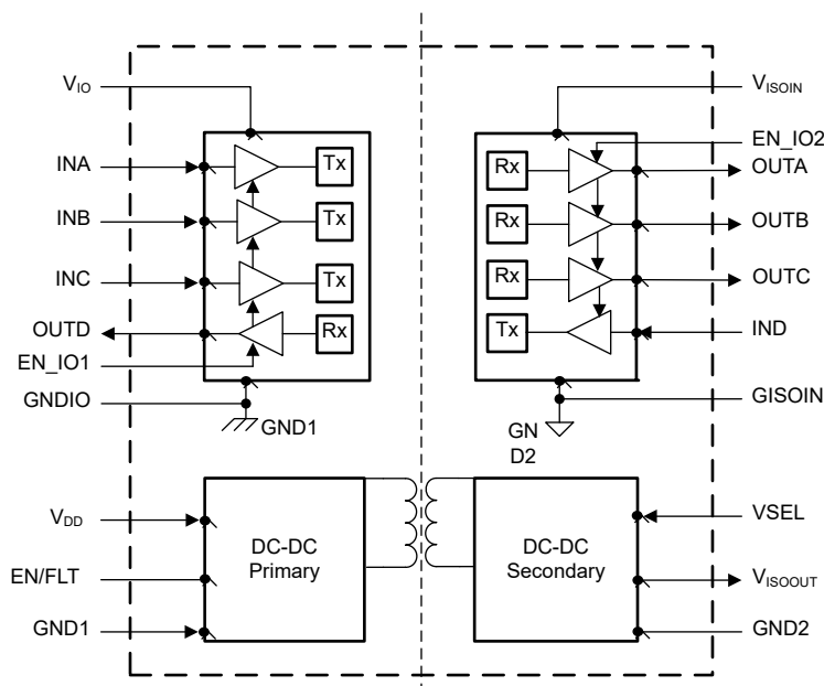
ISOW7741-Q1 简化原理图
