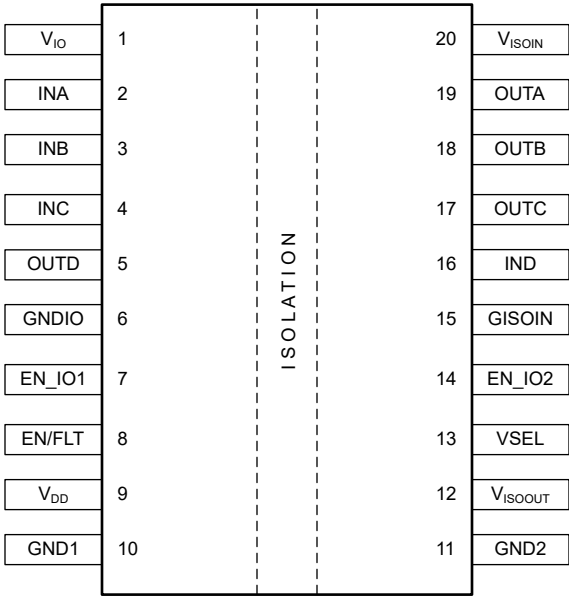
图 4-1. ISOW7741-Q1 DFM 封装 20 引脚 SOIC-WB 顶视图
