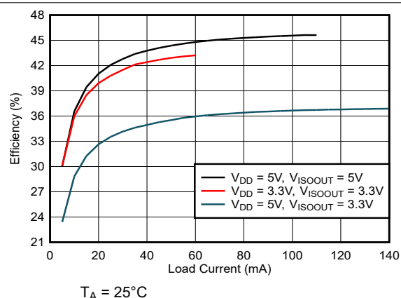
图 5-6. 效率与负载电流 ( I_{ISOOUT} ) 间的关系
