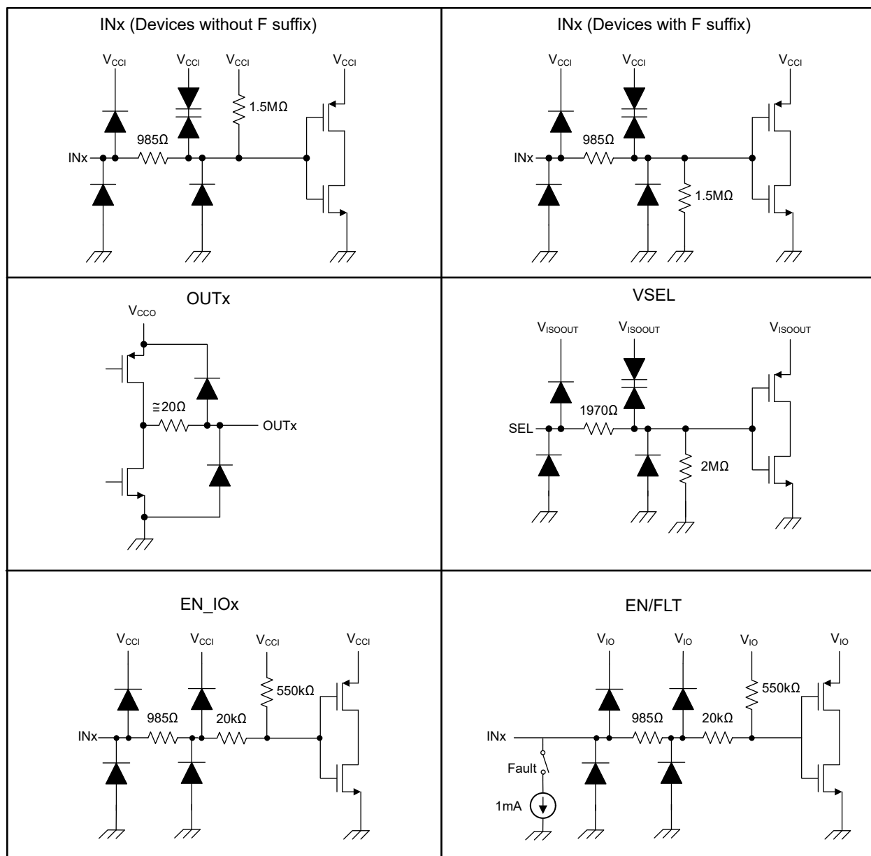
图 7-5. 器件 I/O 原理图
