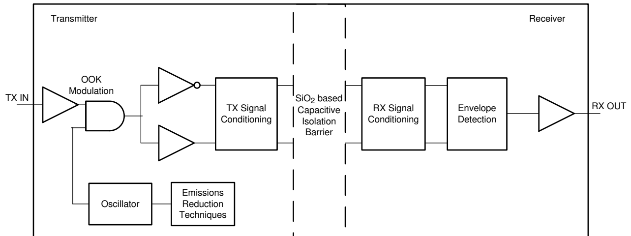
图 7-2. 电容数据通道的概念方框图
