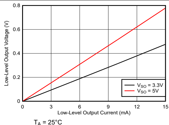
图 5-18. 低电平输出电压与低电平输出电流间的关系
