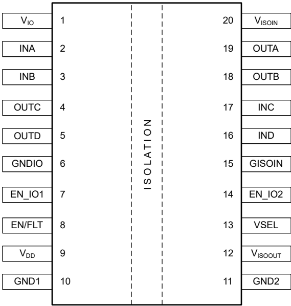
图 4-2. ISOW7742-Q1 DFM 封装 20 引脚 SOIC-WB 顶视图
