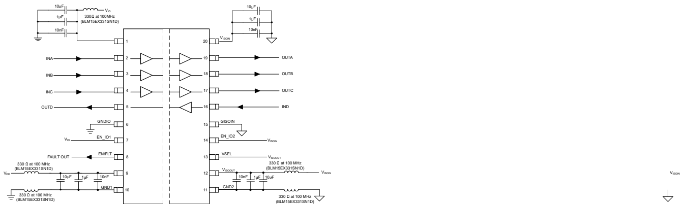
图 8-2. 典型 ISOW7741-Q1 电路组装
