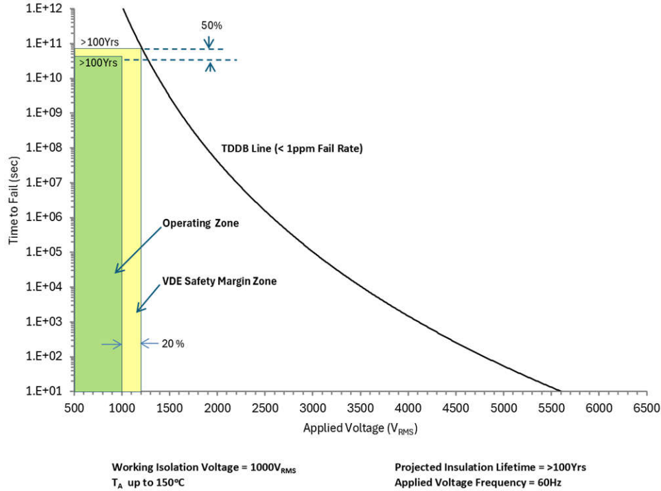
图 8-6. 绝缘寿命预测数据
