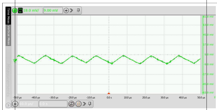
图 5-27. 5V 下使用 10\mu F 电容器和 110mA 负载时的 V_{ISOOUT} 纹波电压
