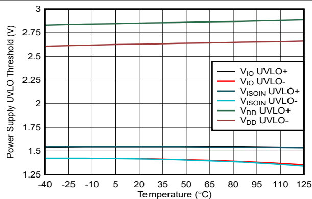
图 5-15. 电源欠压阈值与自然通风条件下的温度间的关系
