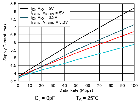
图 5-14. ISOW7742-Q1 通道电源电流与 CL = 0pF 时的数据速率间的关系
