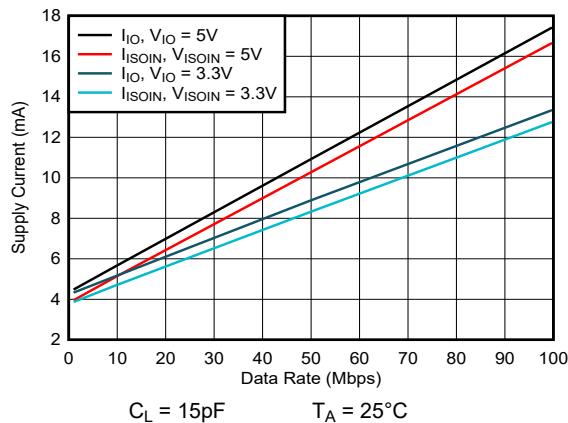
图 5-13. ISOW7742-Q1 通道电源电流与 CL = 15pF 时的数据速率间的关系
