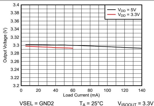
图 5-3. 隔离式电源电压 ( V_{ISOOUT} ) 与负载电流 ( I_{ISOOUT} ) 间的关系
