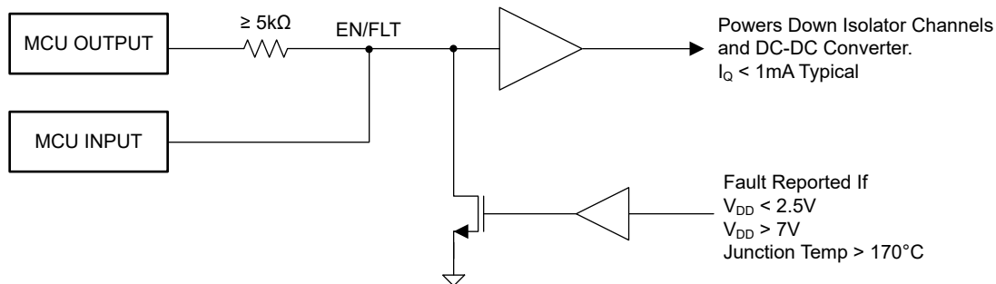
图 7-4. EN/FLT 故障引脚图
