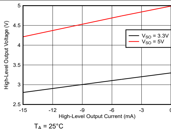
图 5-17. 高电平输出电压与高电平输出电流间的关系
