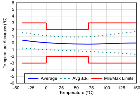
图 6-1. 精度与温度间的关系
