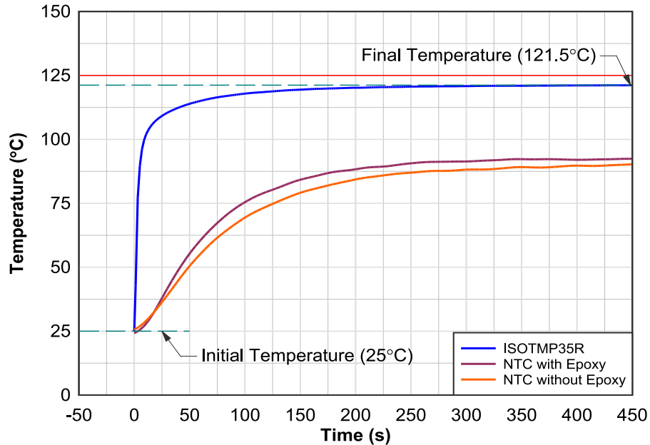
图 7-10. 热响应比较
