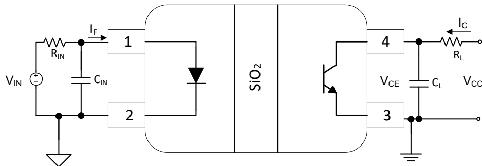
图 7-4. ISOM811[0-3]-Q1 带宽测试电路
