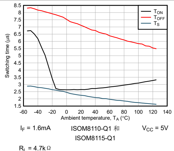
图 6-30. 开关温度与环境温度间的关系
