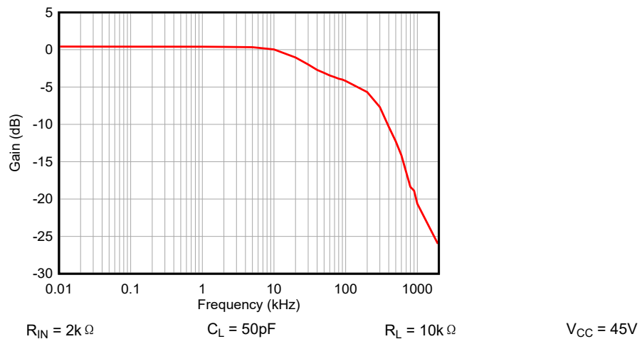
图 9-6. R_L = 10k\Omega 时的带宽
