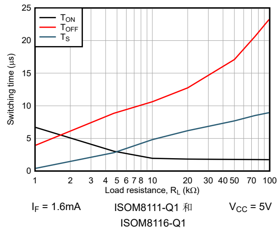
图 6-27. 开关时间与负载电阻间的关系
