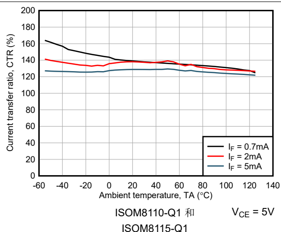
图 6-22. 电流传输比与环境温度间的关系
