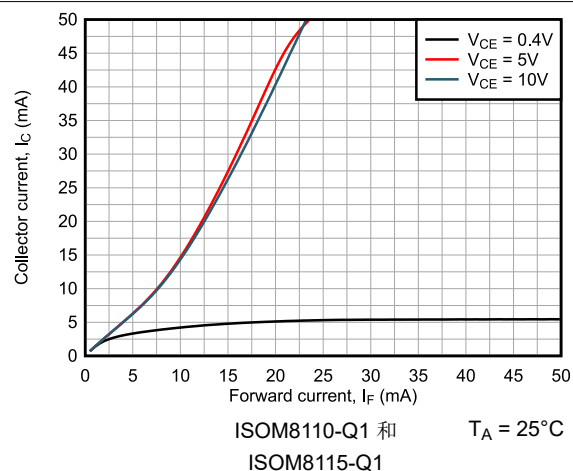
图 6-10. 集电极电流与正向电流间的关系
