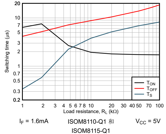
图 6-26. 开关时间与负载电阻间的关系
