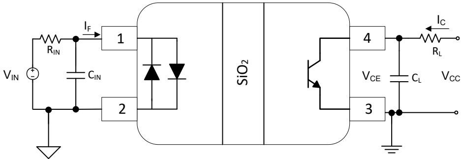
图 7-5. ISOM811[5-8]-Q1 带宽测试电路
