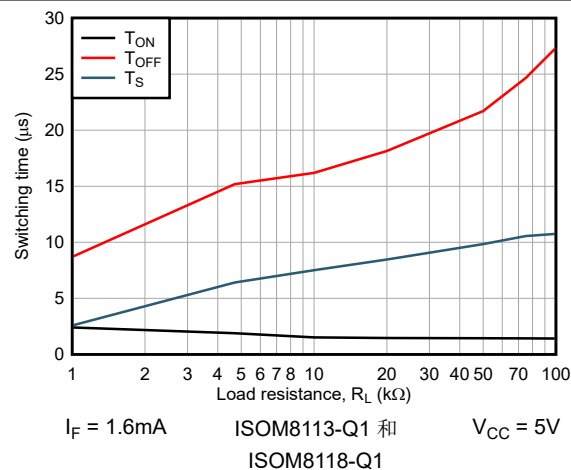
图 6-29. 开关时间与负载电阻间的关系
