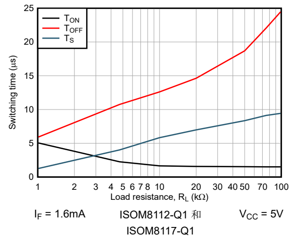
图 6-28. 开关时间与负载电阻间的关系
