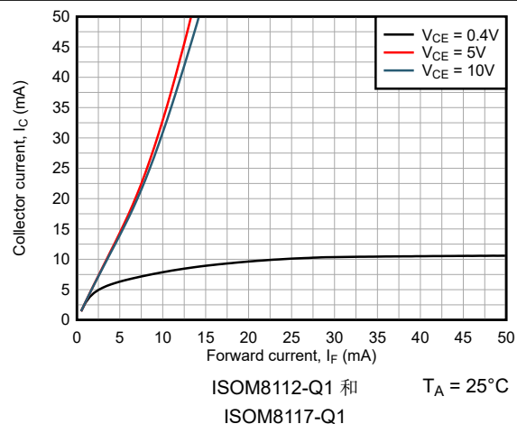
图 6-12. 集电极电流与正向电流间的关系
