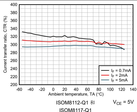
图 6-24. 电流传输比与环境温度间的关系
