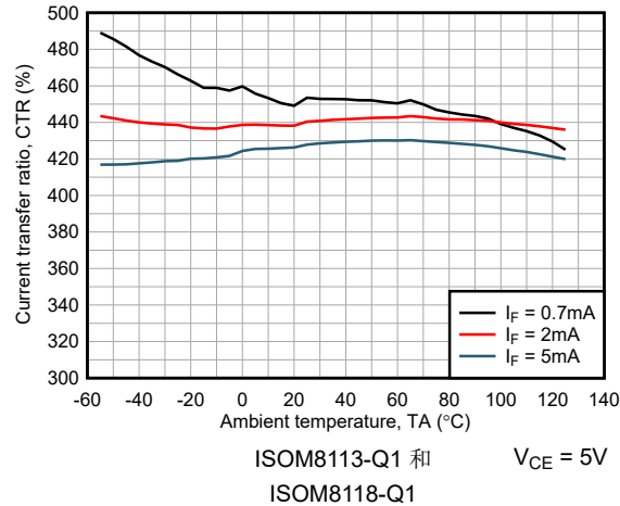
图 6-25. 电流传输比与环境温度间的关系
