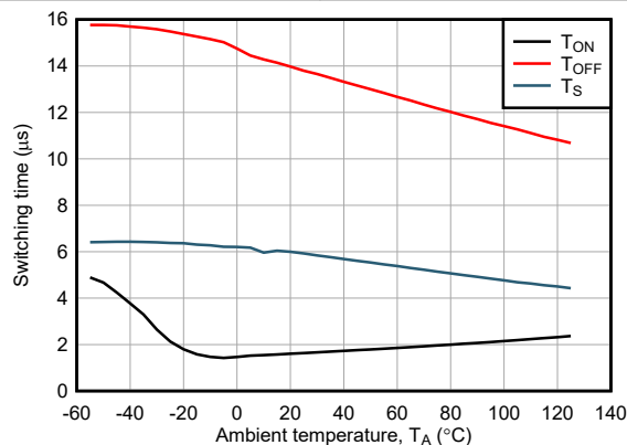
图 6-31. 开关时间与环境温度间的关系
