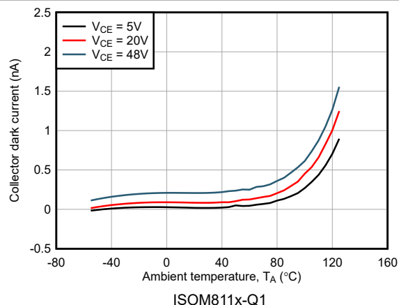
图 6-8. 集电极暗电流与环境温度间的关系
