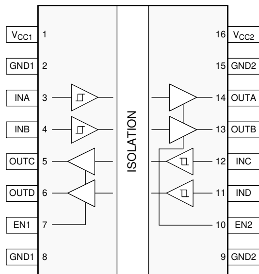
图 4-1. DW 和 DWW 封装 16 引脚 SOIC 俯视图
