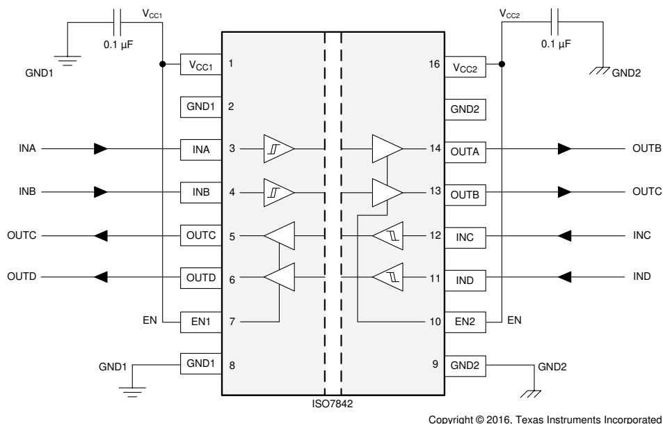
图 8-2. 典型 ISO7842 电路组装
