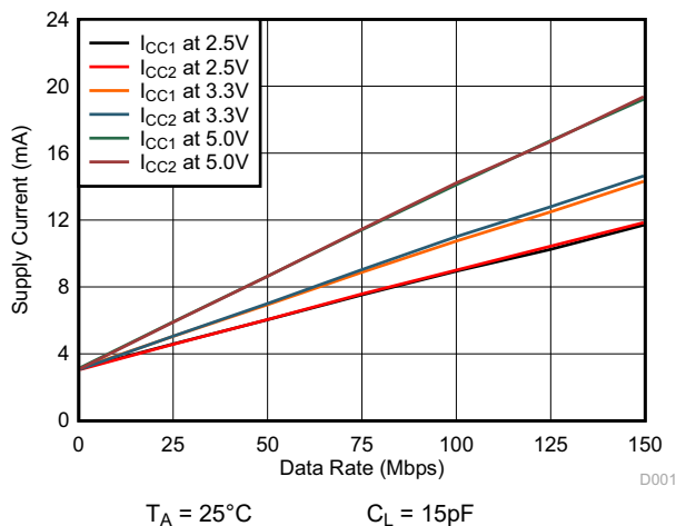
图 5-5. 电源电流与数据速率之间的关系 (15pF 负载)
