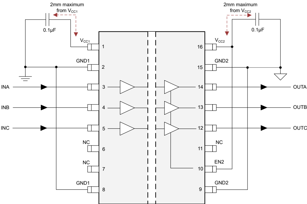
图 8-2. 典型 ISO7830 电路组装
