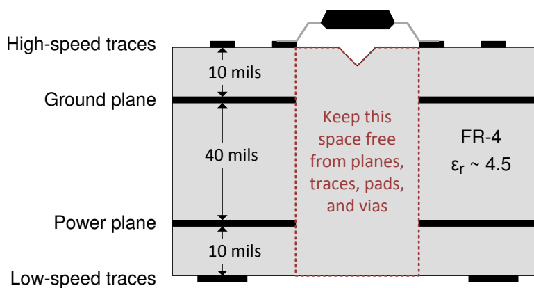
图 8-4. Layout Example
